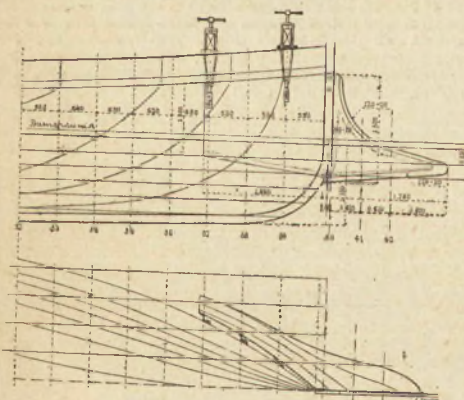
Фиг. 3. Ледокольный плугъ.
