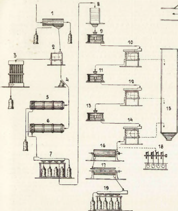
Фиг. 1. Схема выработки пшениной крупы.
