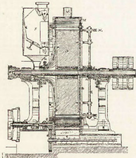
Фиг. 6. Продольный разрезъ.
