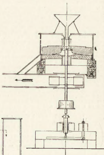
Фиг. 2. Разрѣзъ просорушного постава.
