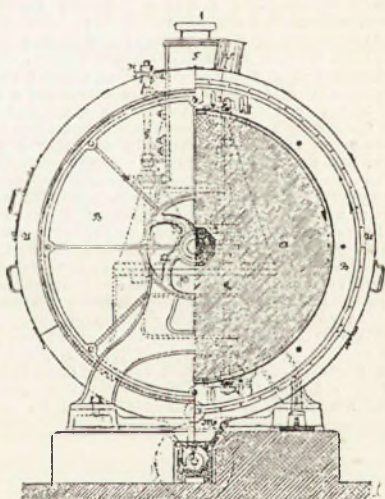
Фиг. 7. Поперечный разрезъ.
