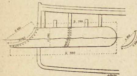
Фиг. 2. Ледокольный плугъ.
