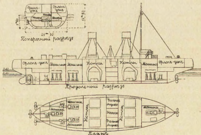
Фиг. 1. Ледоколъ „Ермакъ“. Разрѣзы и планъ.
