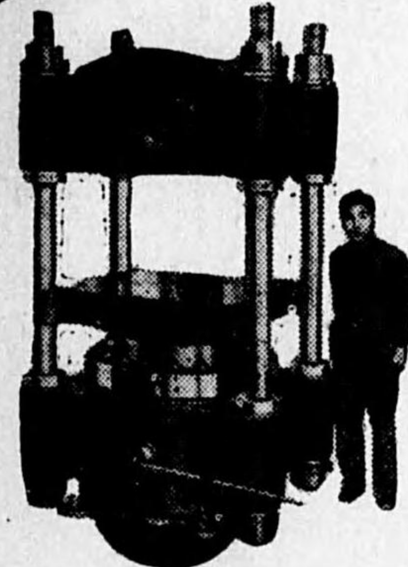
(500噸) 水壓機
