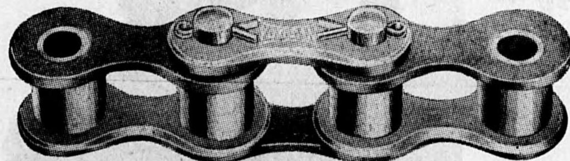
傳導用及機關車用ローラーチェーン
