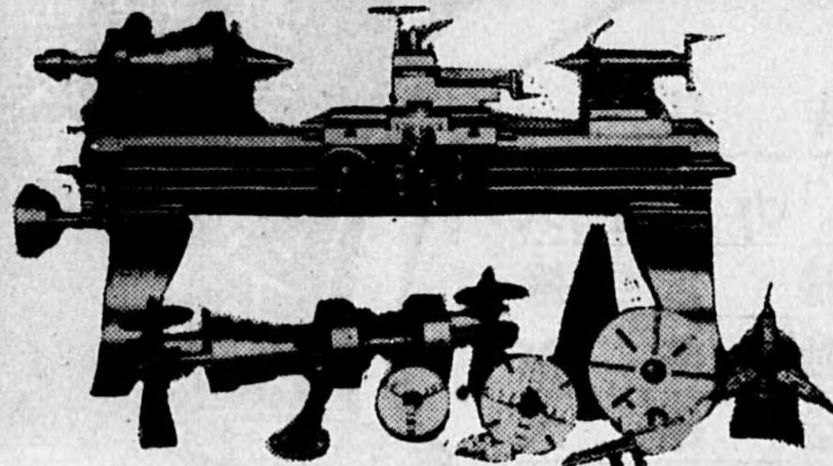
米式六呎旋盤
