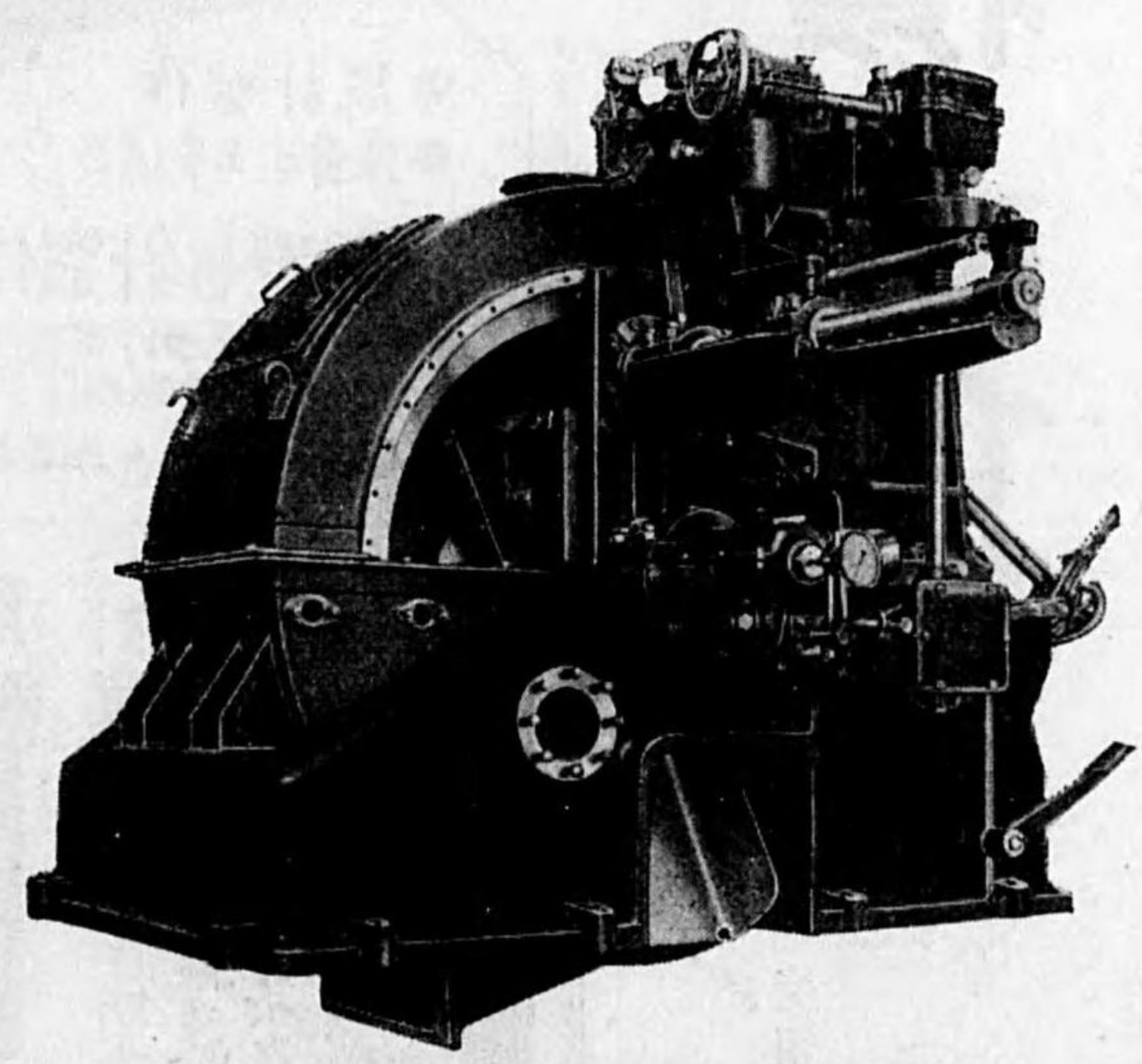
最新型自働取橫式遠心分離機 トツケスバ 一徑米 巾六八
