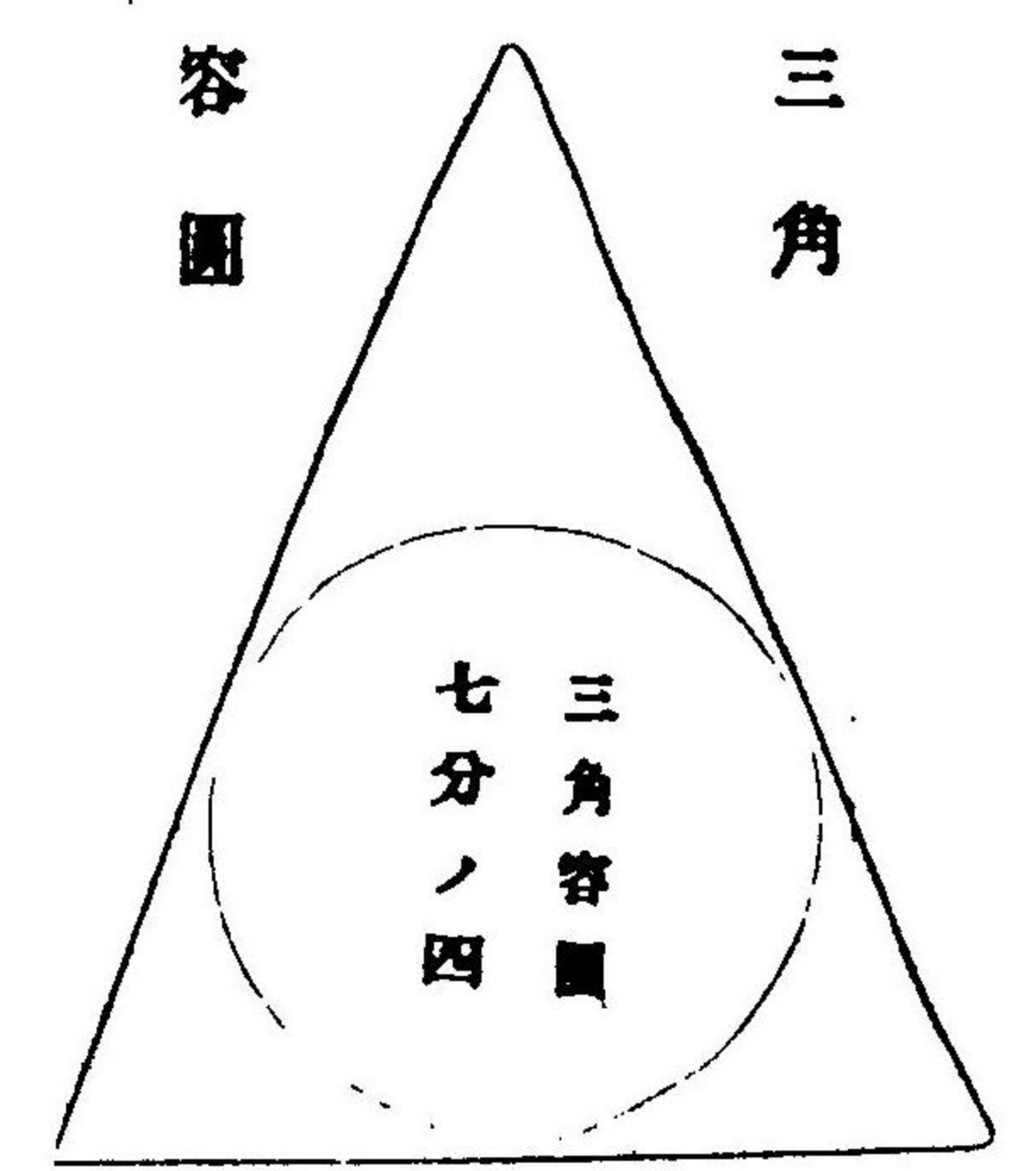
角三容圓
