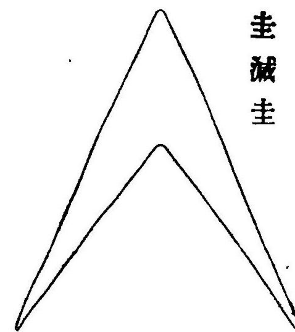
減圭 弧矢
