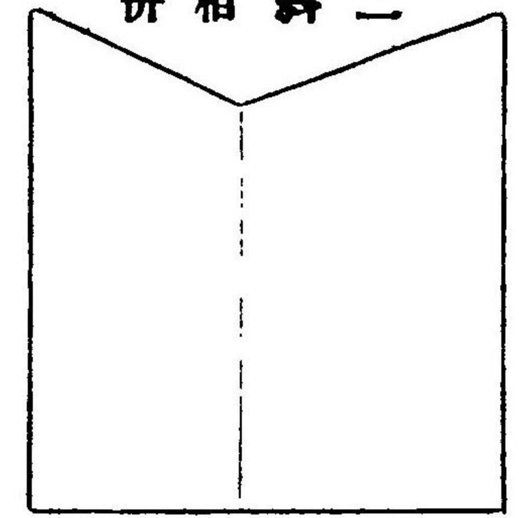
弧併圭二
