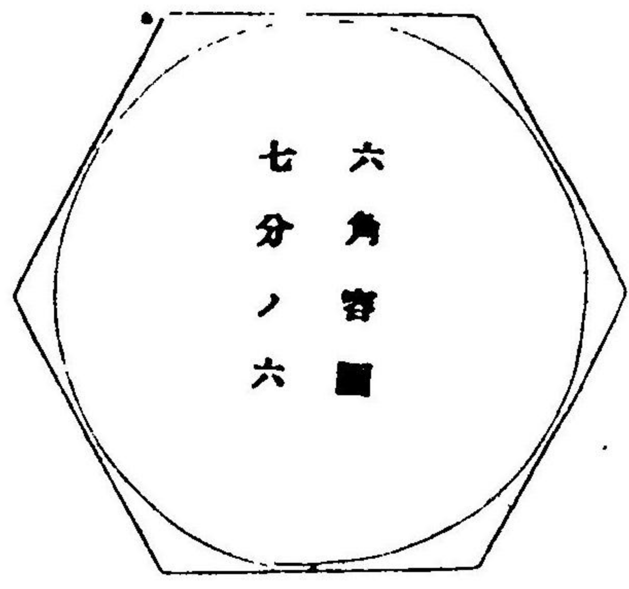
圓容角六
