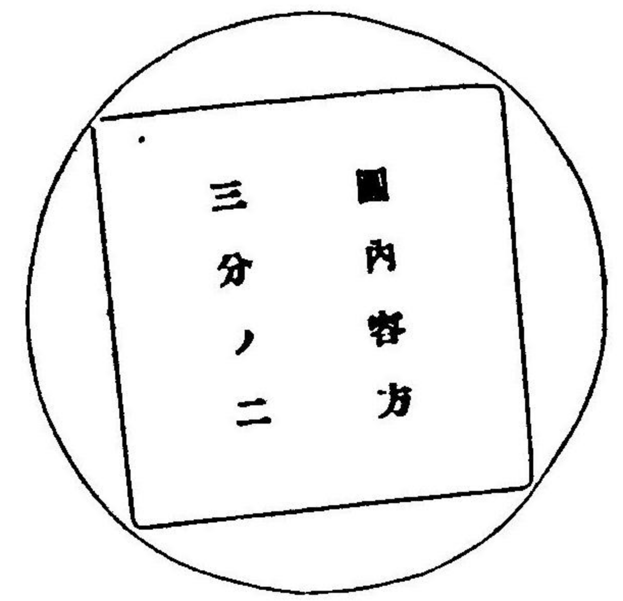
方容内圓
