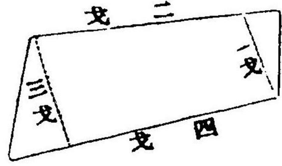
算 截 圭 二
