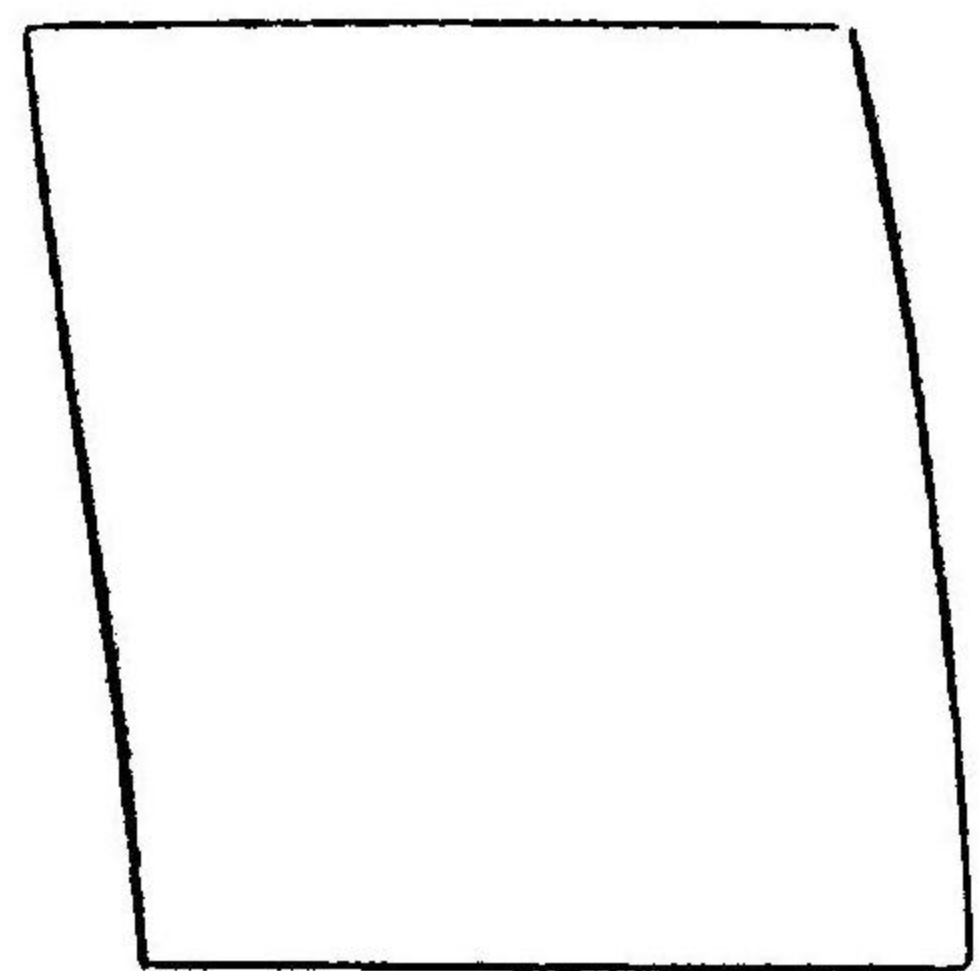
田 斜
