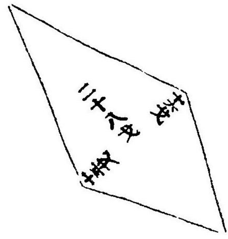
併圭二又
