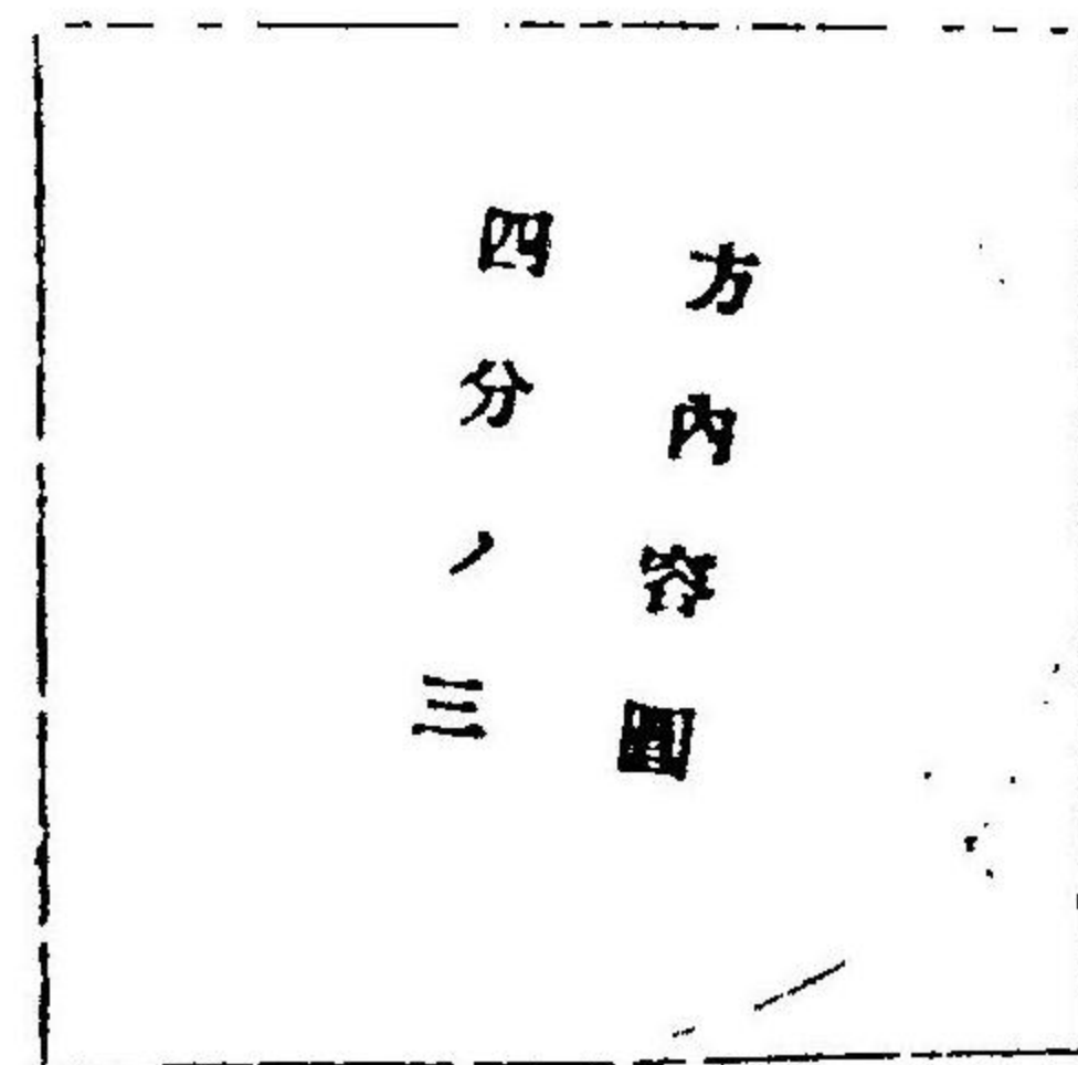
圓容內方
