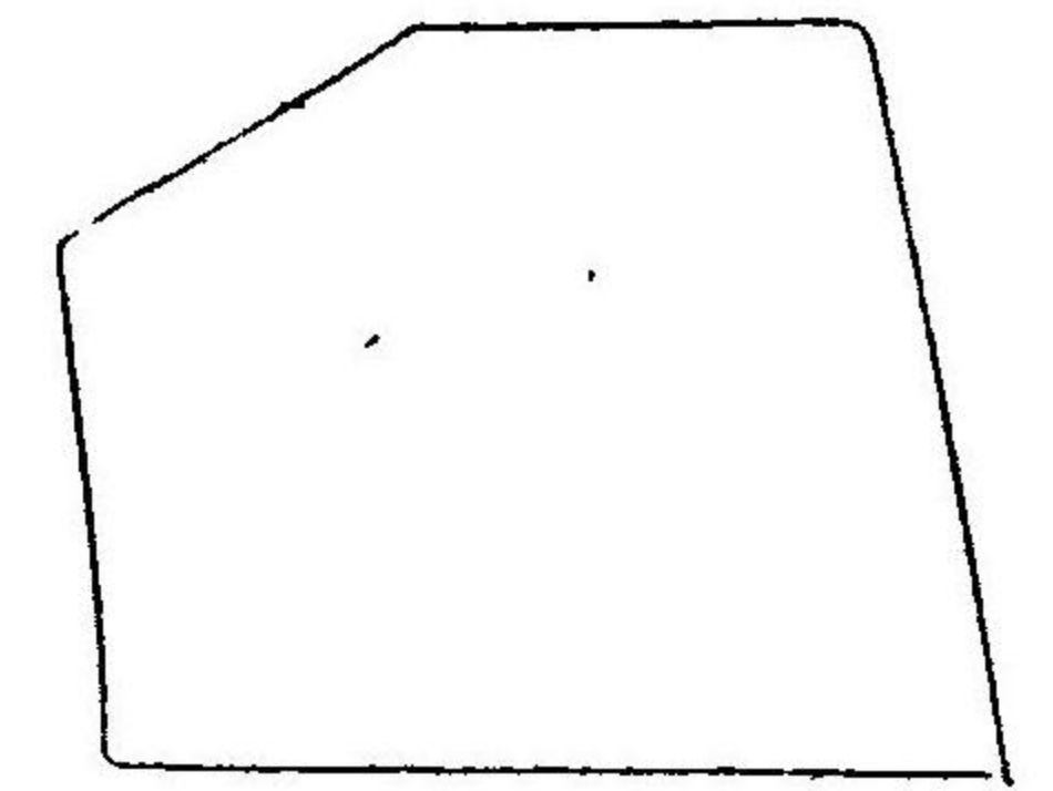
股勾減斜
