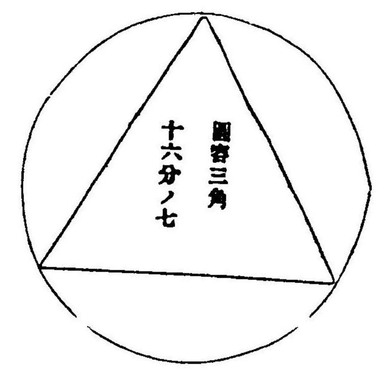
角三容圓
