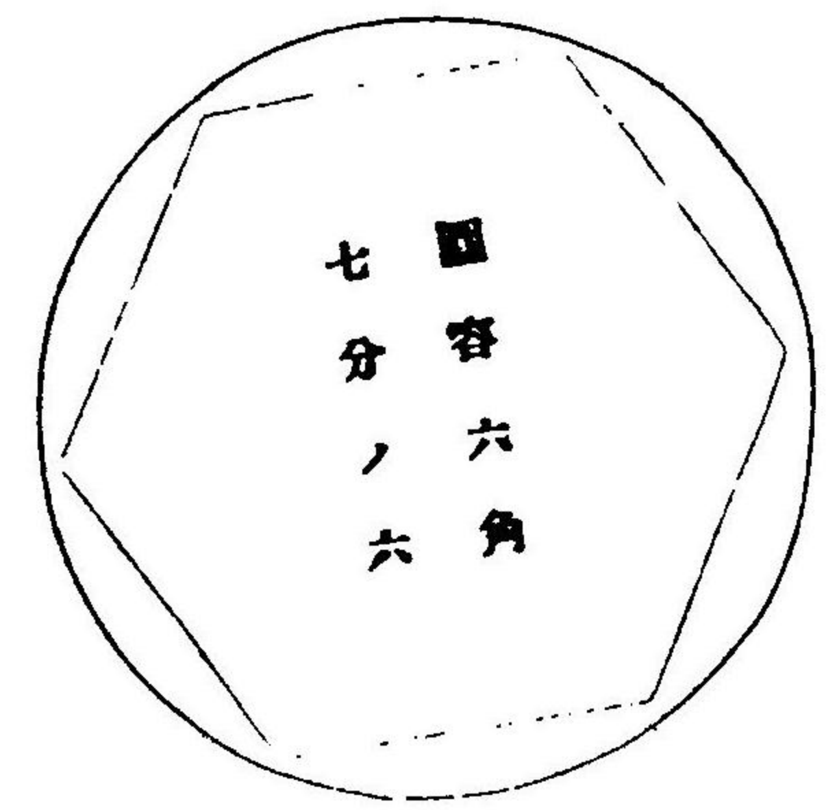
角六容圓
