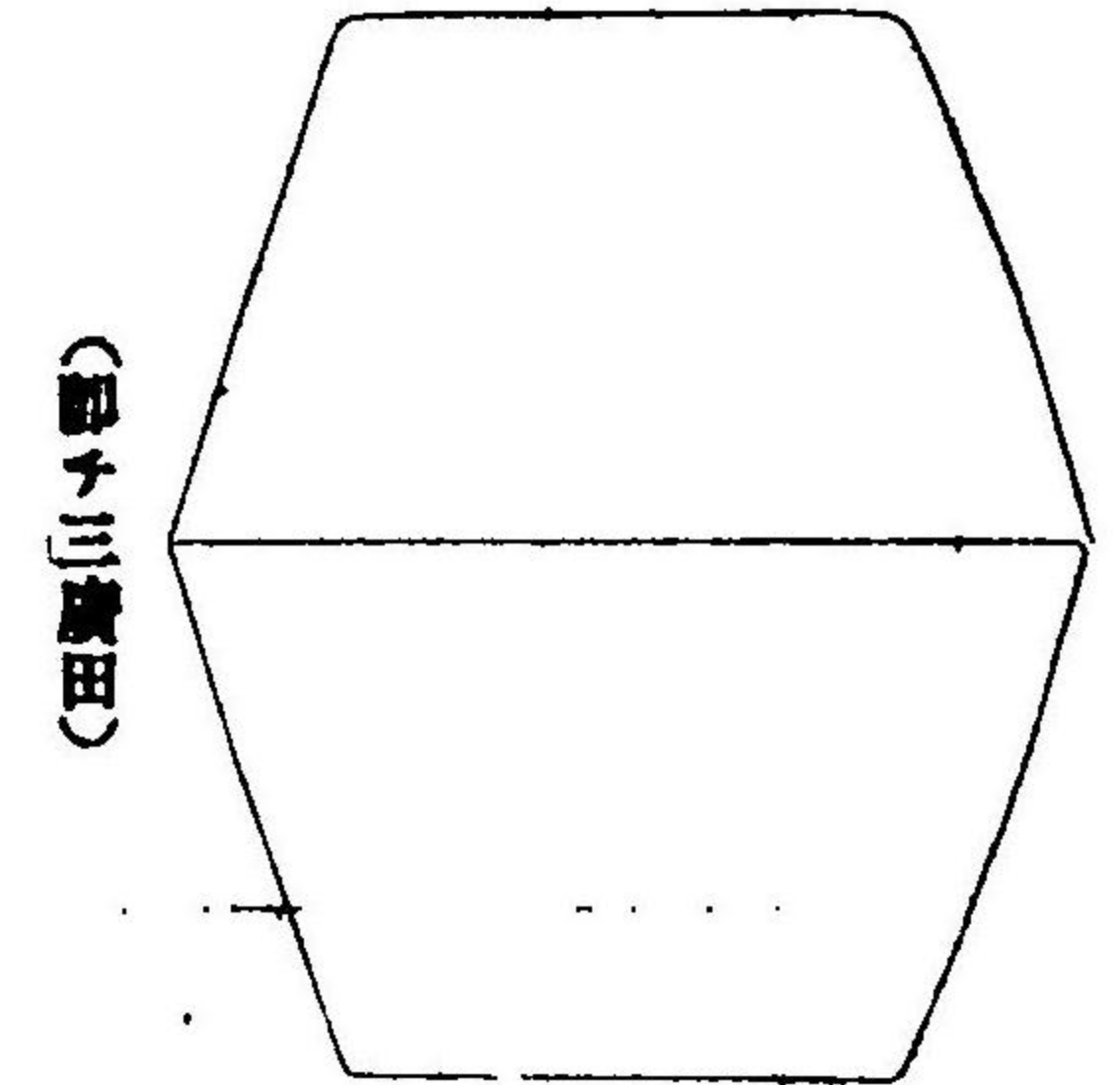
併相斜二
