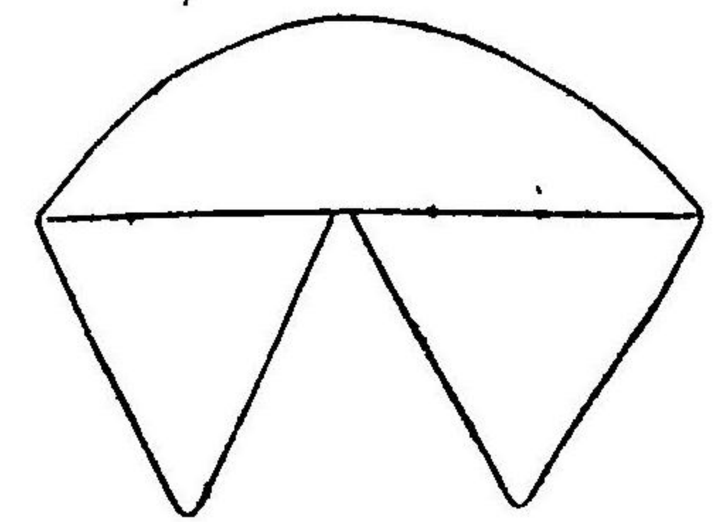
弧併圭二
