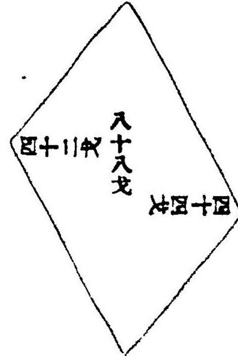
併相圭二
