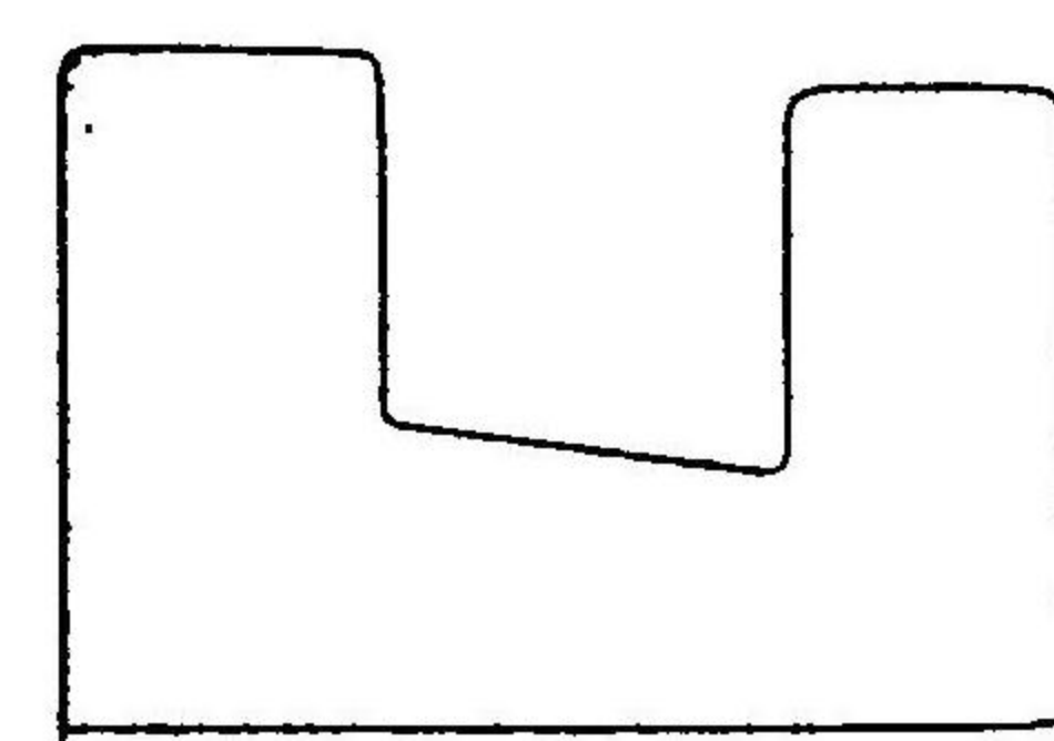
方減田斜
