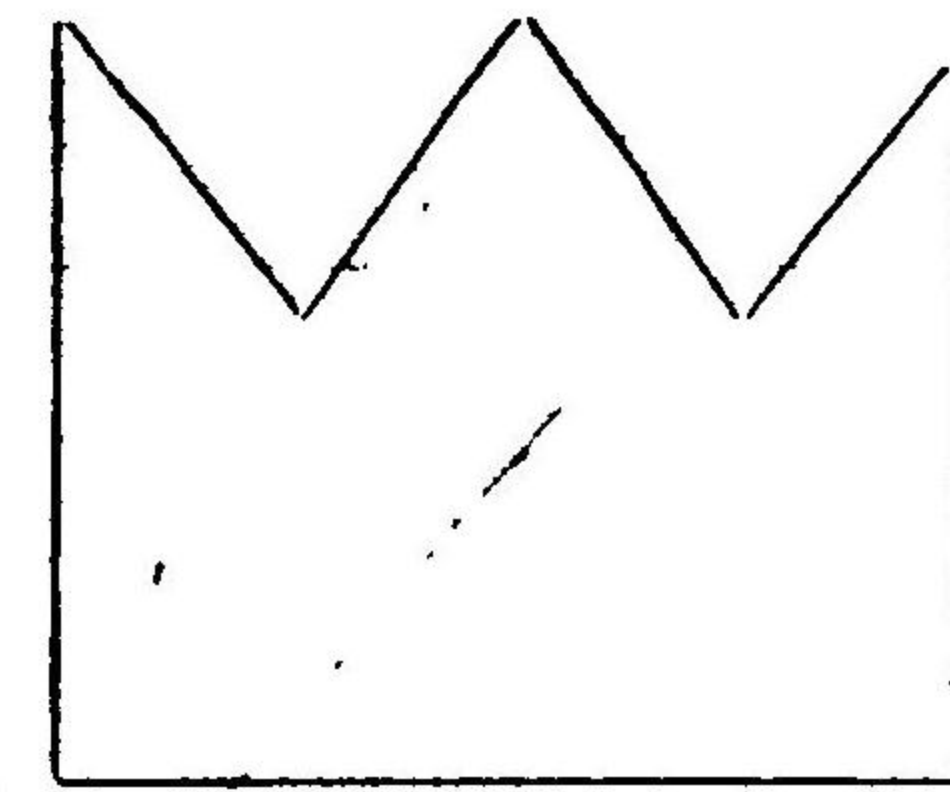
圭二減方
