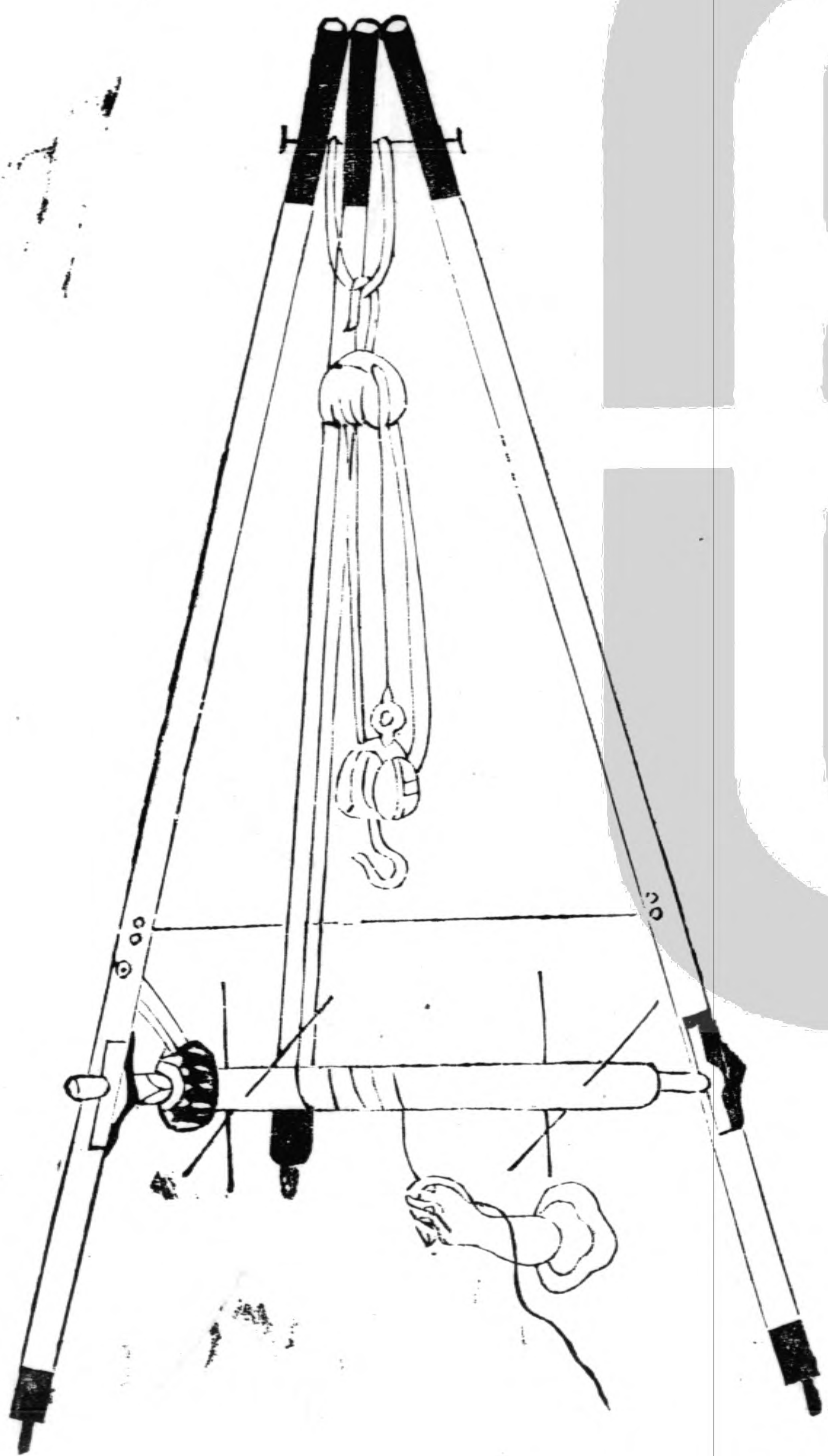
做製西洋舉重滑車絞架圖
