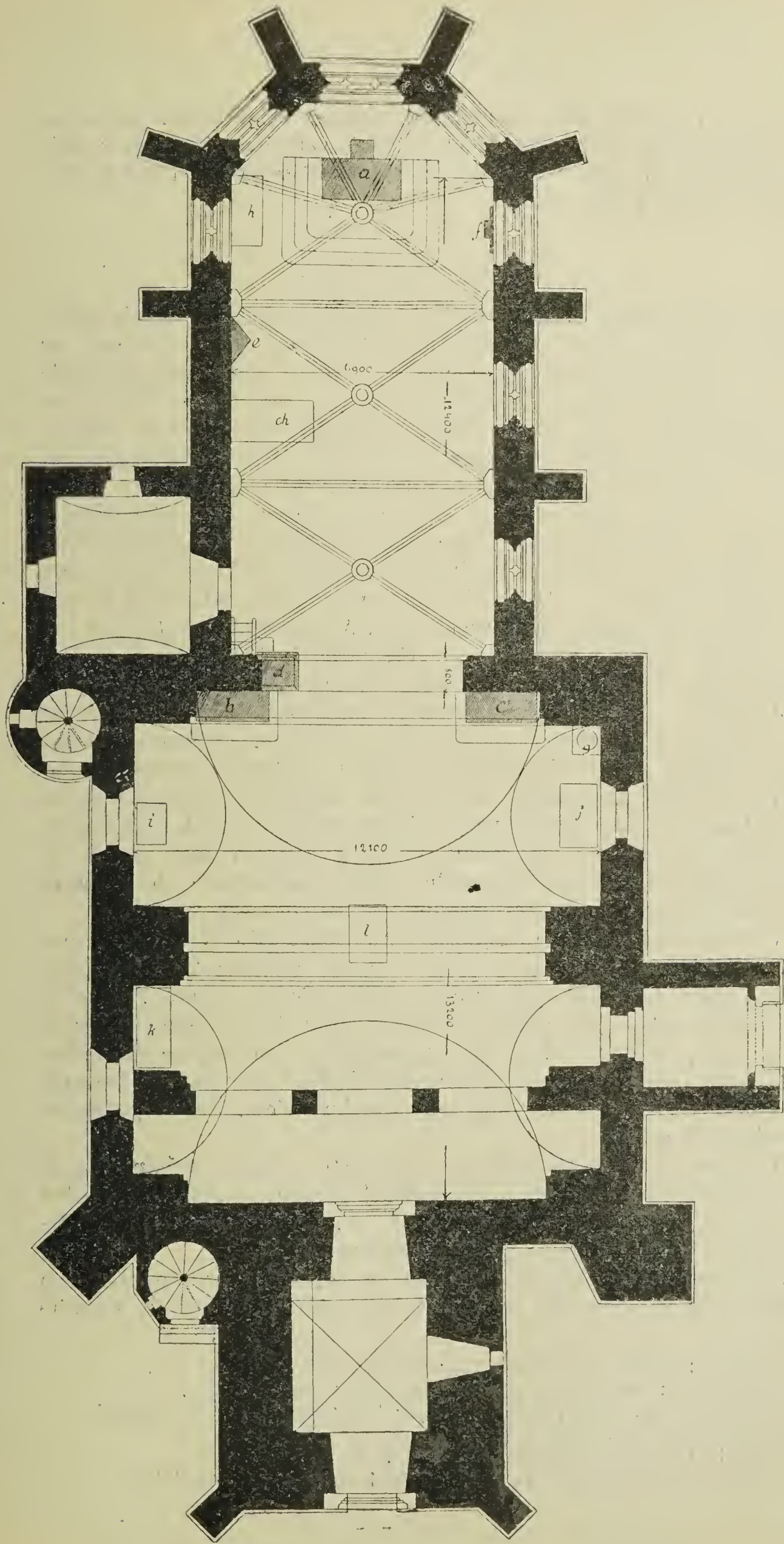
Obr. 12. Půdorys kostela v Charvátci dle návrhu stavitele V. Faigla kreslil F. X. Kodeš. Poměr 1 : 200.
