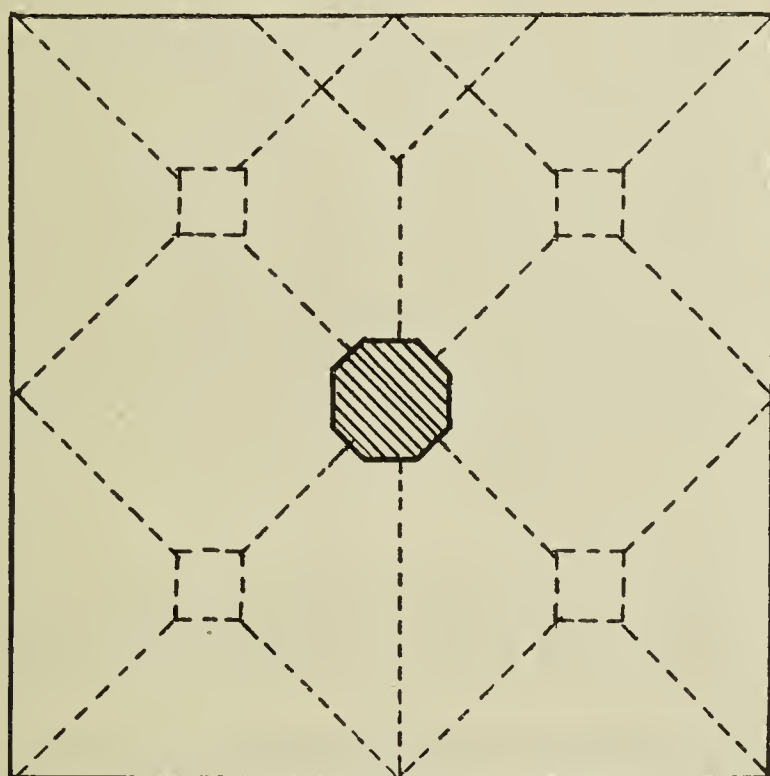
Obr. 3. Síť klenbová v lodi kostela ve Wiese.
