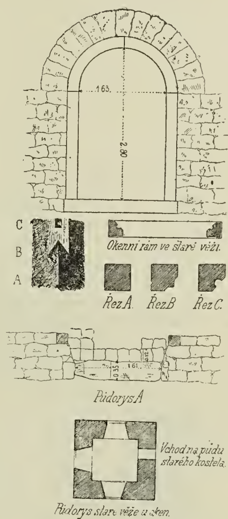
Obr. 2. Půdorys okna staré věže kostelní.
