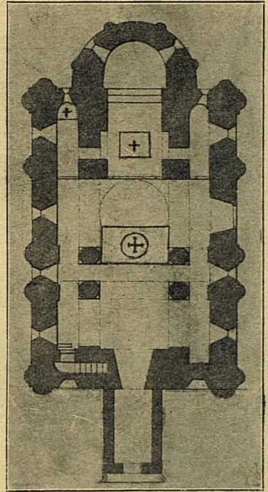
Планъ Храма Спасителя въ Полоцкомъ Спасо-Евфросиніевскомъ м-рѣ,
