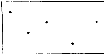
2. Cassiopeia . Pump o ser yn ffurf y llythren W.
