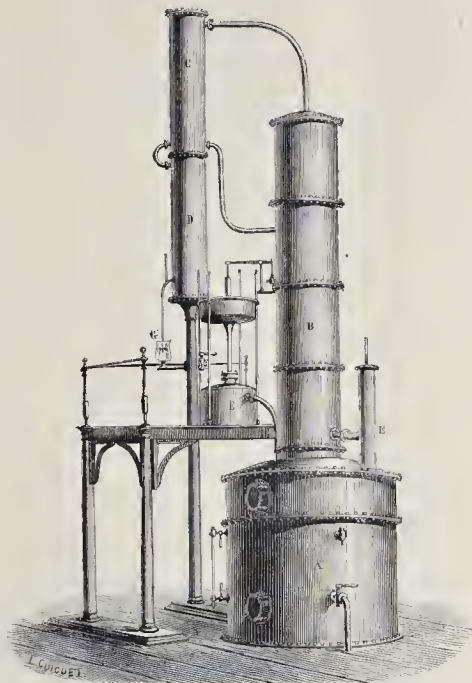
APPAREIL SAVALLE. — Rectification et épuración des alcools. (Médaille d'or.)
