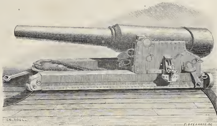
CANON GAUDET. — Dessin de M. Noël.
