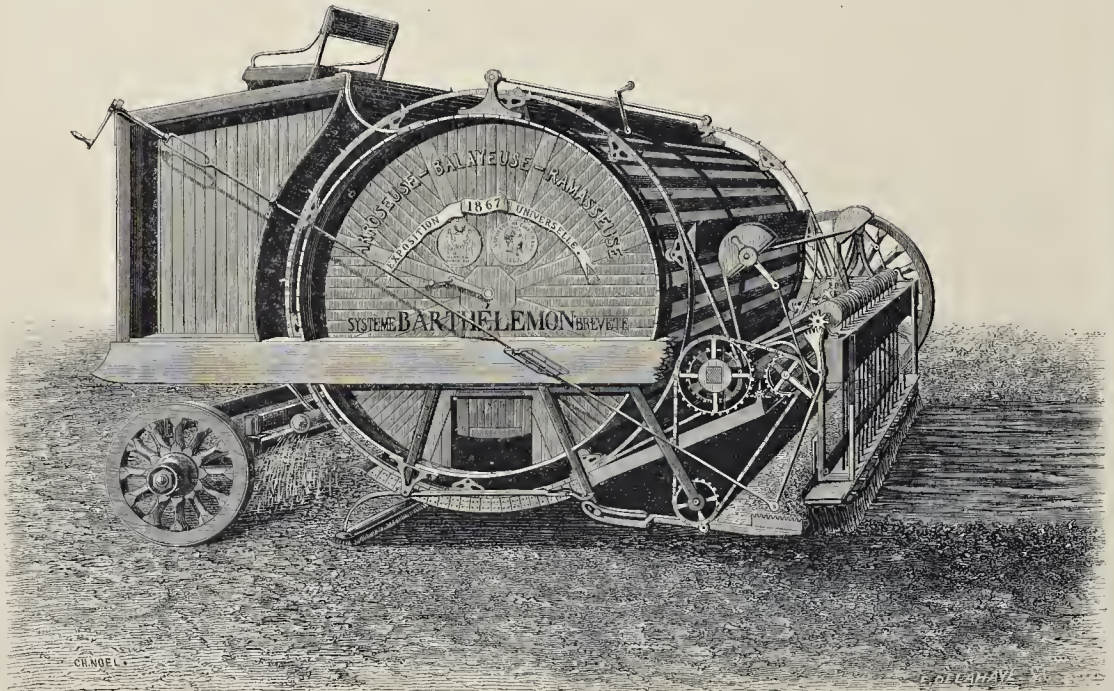
LA BALAYEUSE DE M. BARTHÉLEMON. — Dessin de M. Noël.
