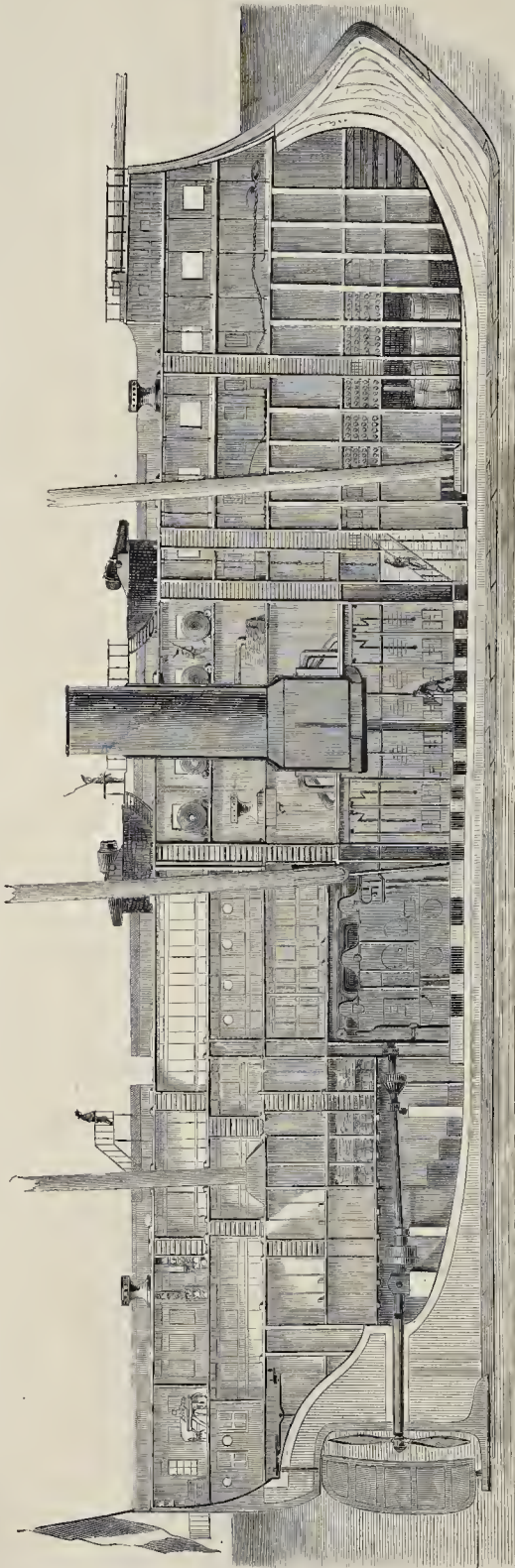
INTÉRIEUR D'UNE FRÉGATE CUIRASSÉE. (Type MARENGO.)
