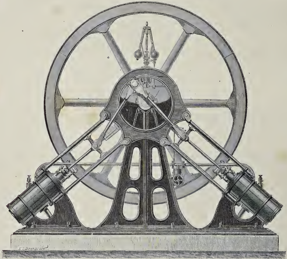
MACHINE A CYLINDRES INCLINÉS DE M. BOURDON.
