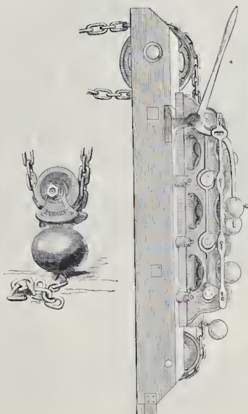
Parachute automatique et guide tendeur de sûreté.
