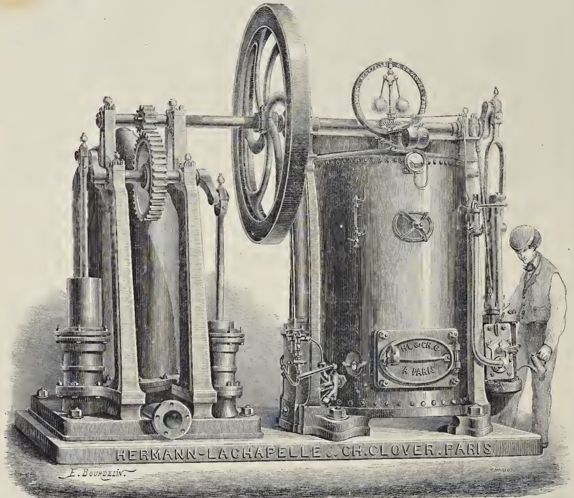
MACHINES DE MM. HERMANN-LACHAPPELLE ET CH. CLOVER.
