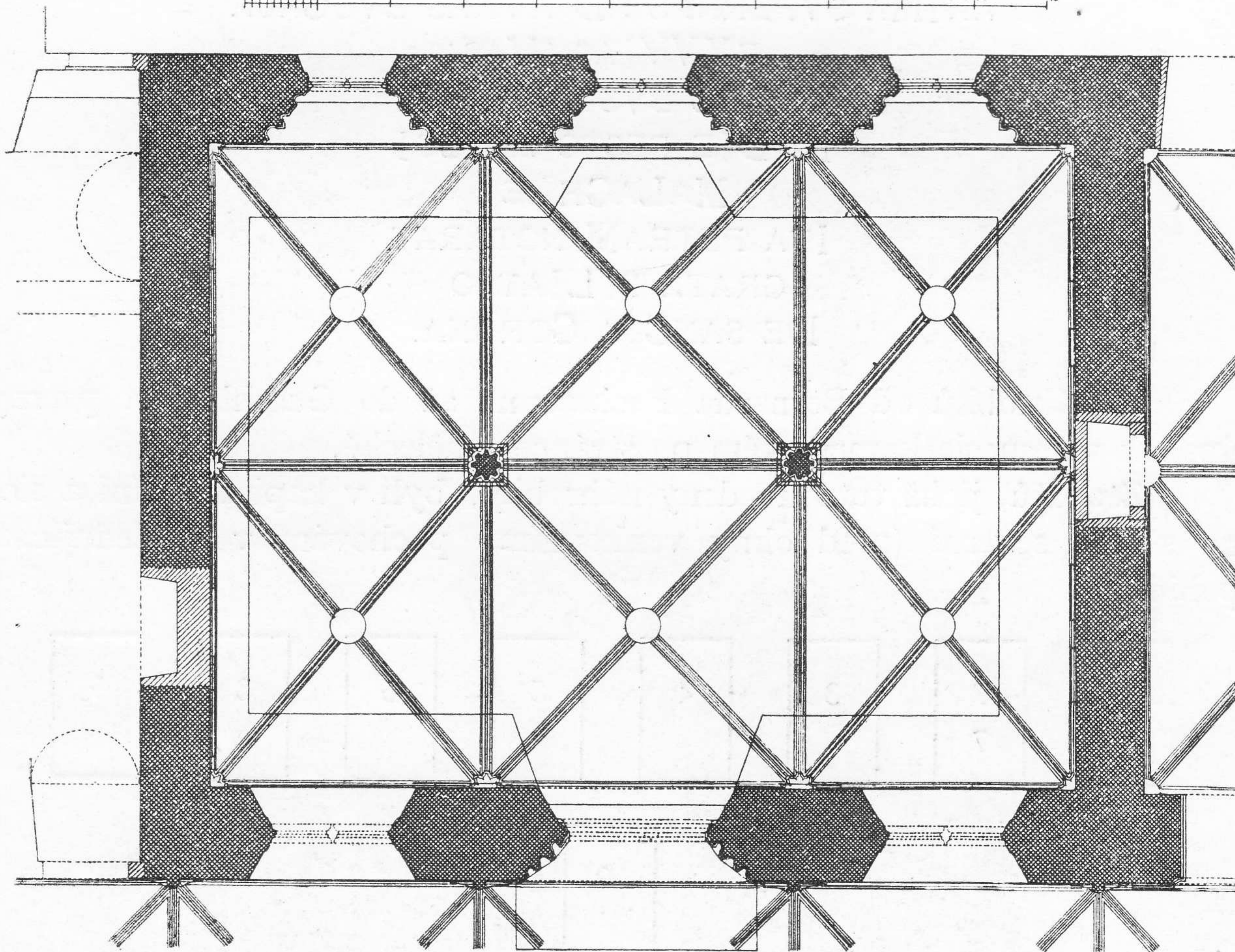
Obr. 188. Zlatá Koruna. Půdorys a profil kapitulní síně.
