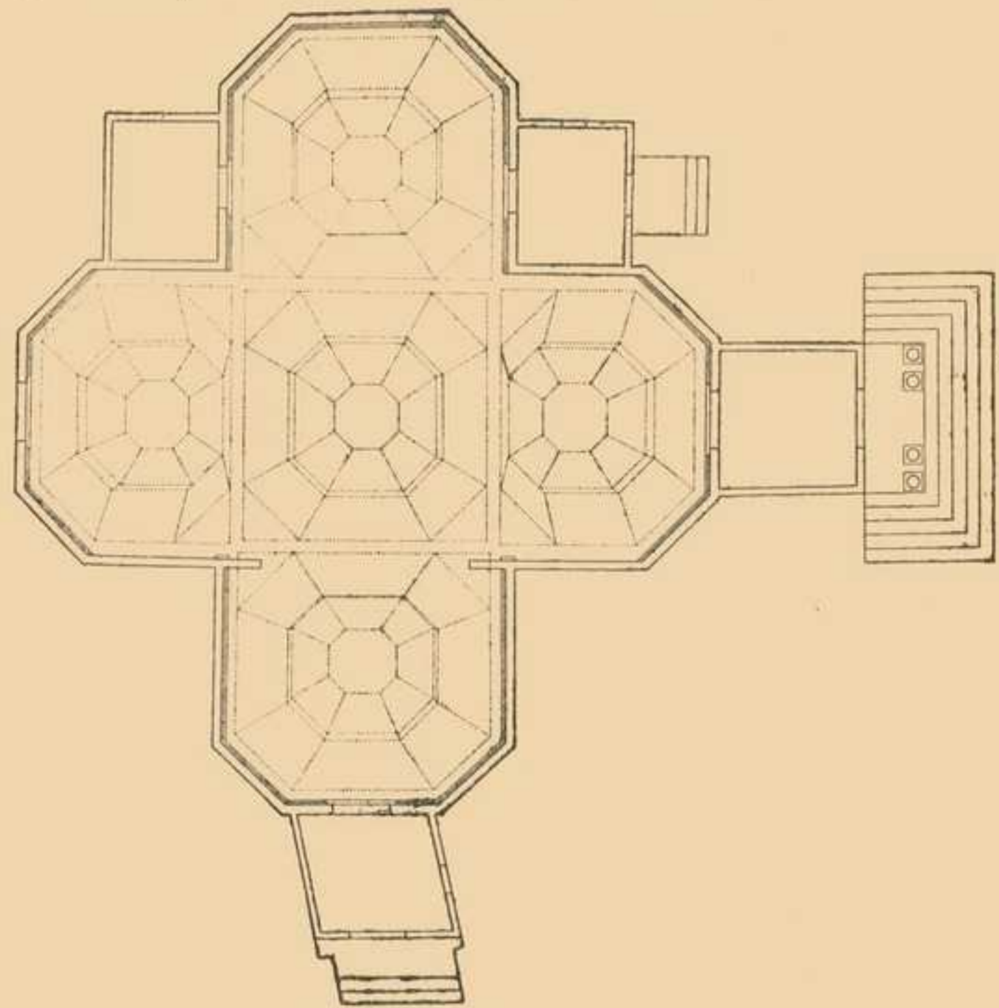
Рис. 2. Планъ Покровской церкви въ г. Ромнахъ.
