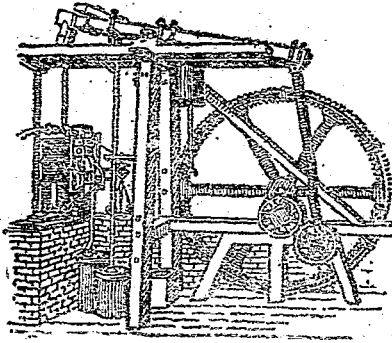
華特第一所發明之蒸汽機
