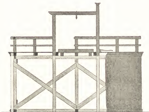
Afb. N o . 370. Het laatste schavot, dat van Amsterdam, breed 9.35 M., diep 5.50 M., hoog 4.25 M., tijdens eene terechtstelling geheel met zwart laken omkleed 2) .
