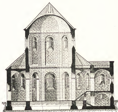
Afb. N o . 181. Sint-Walburgskerk te Groningen, in doorsnede.
