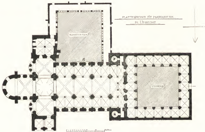
Afb. N o . 197. Plattegrond der gewezen Mariakerk te Utrecht.
