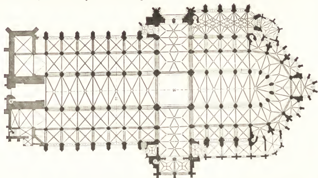
Afb. N o . 161. Sint-Jan te 's-Hertogenbosch, gebouwd in de jaren 1419—1519.
