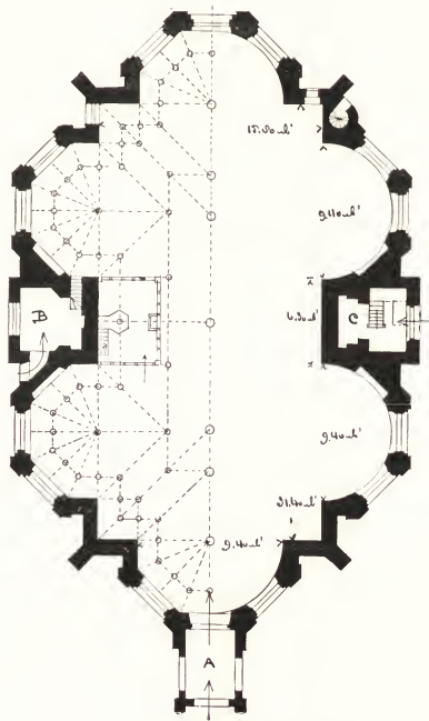
Afb. N o . 252. Plattegrond der Nieuwe Kerk op het Spui te 's Gravenhage.
