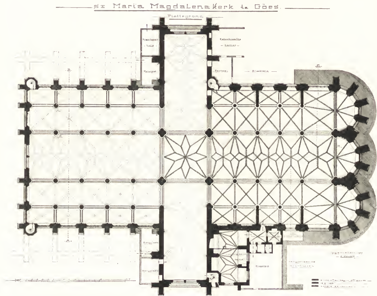
Afb. N o . 220. Plattegrond der onvoltooid gebleven kerk, voór zooveel zij, ná haren brand op 11 Sept. 1618, herbouwd werd.
