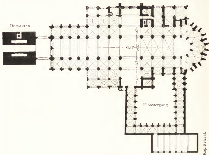
Afb. N o . 165. De onvoltooide Dom of Sint-Maartenskerk te Utrecht zoals zij was tot Augustus 1674.
