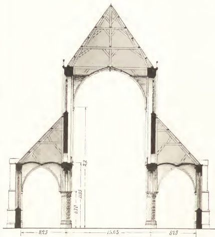
Afb. N o . 168. Sint-Bavo te Haarlem.
