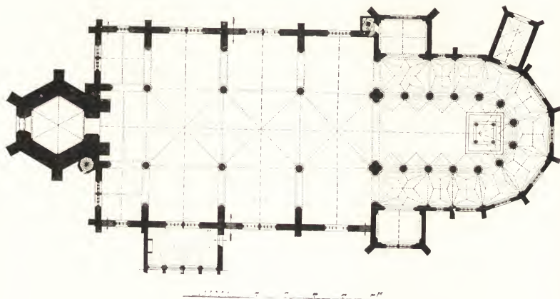
Afb. N o . 217. Overwelfingsplan der Sint-Jacobskerk te 's Gravenhage.
