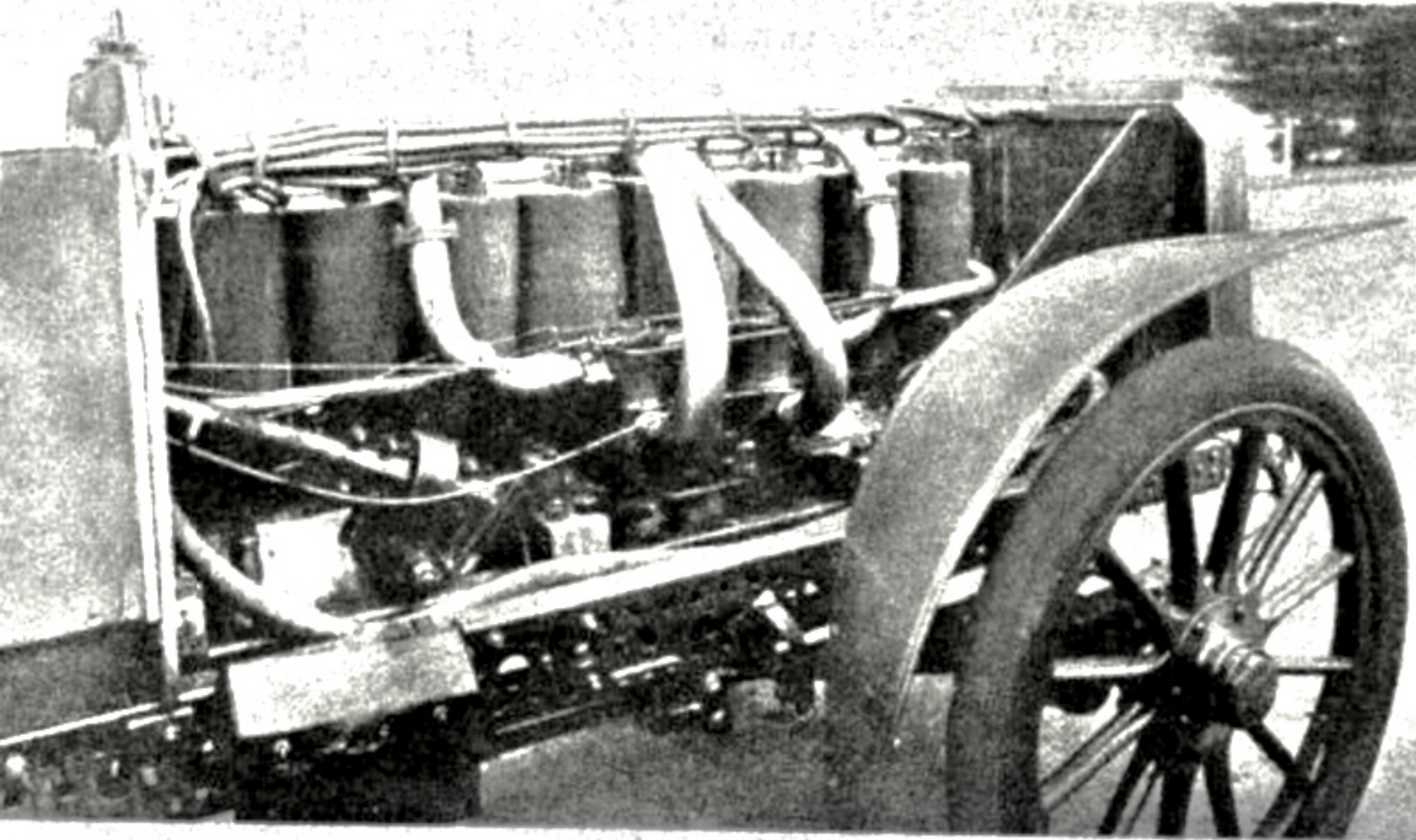
Der Achtzylinder-Motor des 200 PS Bellamywagens.
