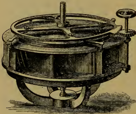
Van de Water Wheel.
