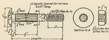
FIG. 3. BOLT AND NUT.
