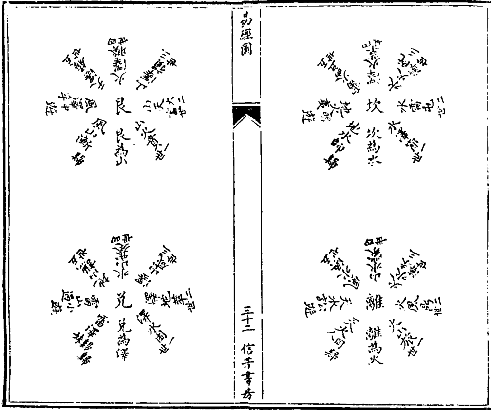
八卦因重圖
