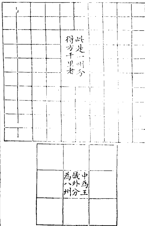
王畿九州圖
