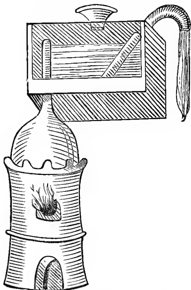
FIG. 4.—Porta's Apparatus, A. D. 1601.
