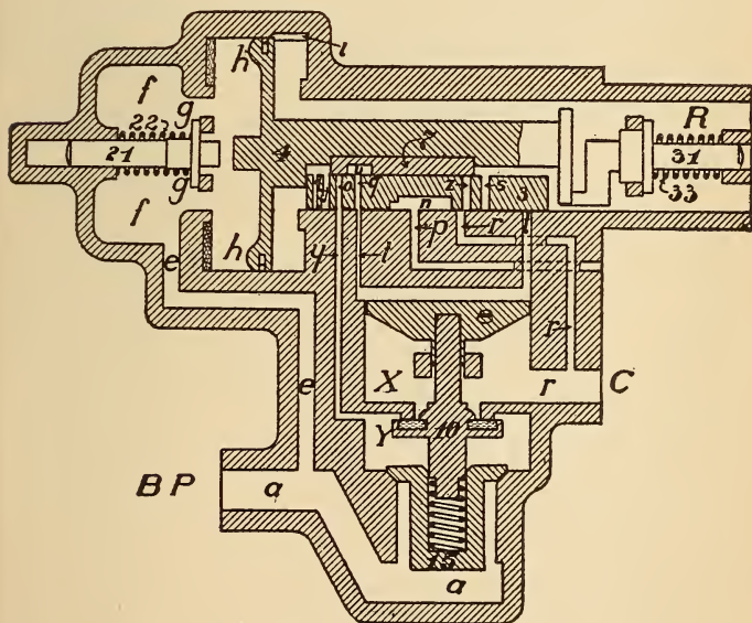
FIG. 329. LAP POSITION
