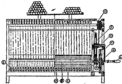
餘姚紡紗機說明圖
