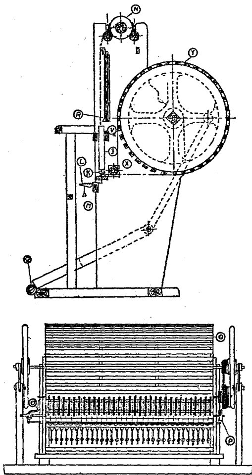
七七紡紗機說明圖
