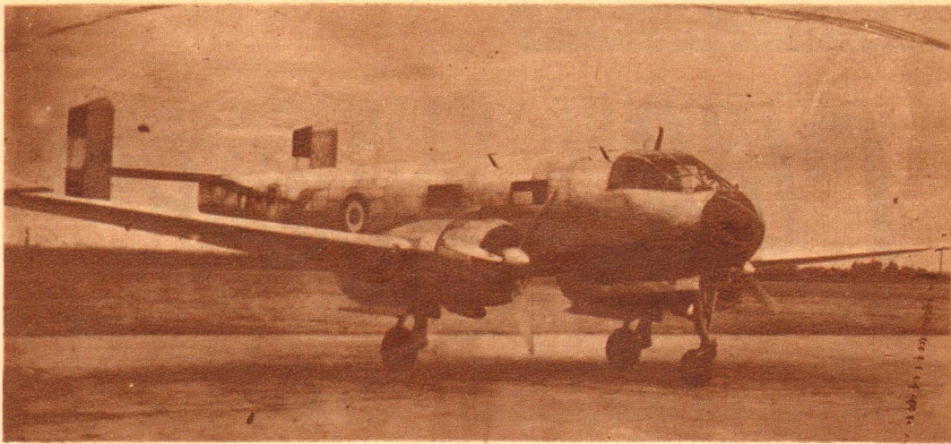
Orgullo de técnica y realización, este avión argentino, de uso múltiple, prototipo I.A.35, totalmente construido por Industrias Aeronáuticas Mecánicas del Estado, unifica en su perfección material la aplicación práctica de los más modernos transportes.
