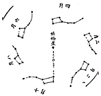
北斗周年迴轉圖 每日下午九時 北斗在天之象
