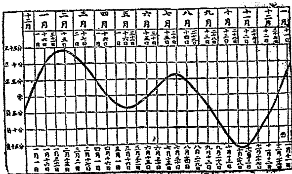
時差曲線圖
