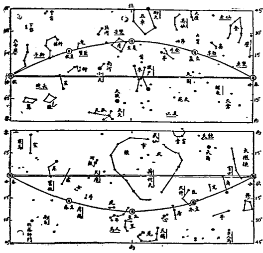
太陽周年躔度圖 圖中雙線為赤道曲線為黃道黃道上下兩圈為太陽 星宿名旁無直畫者為中國原名有直畫者為譯名
