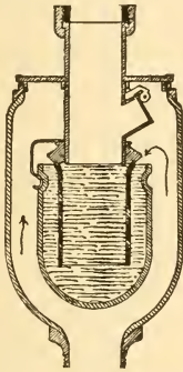
Fig. 91. Air Vent Trap.
