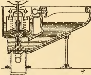
Fig. 389. Plunger Closet.
