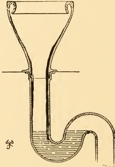
Fig. 407. Long Hopper.
