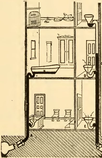
Fig. 239. Trap Siphoning.*
