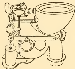
Fig. 388. Plunger Closet.
