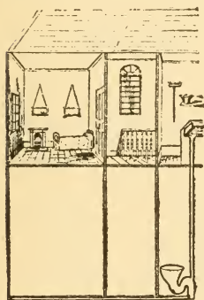
Fig. 629. Untrapped sink waste.
