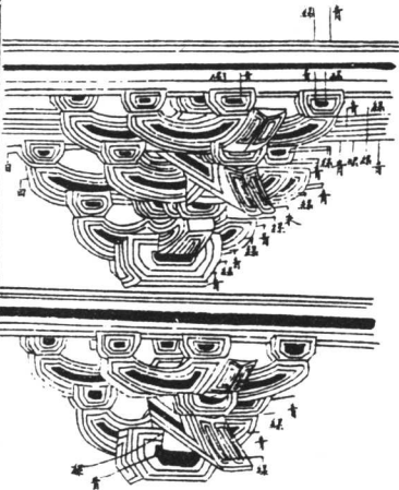
三臺帶紅校間裝名件第十四
