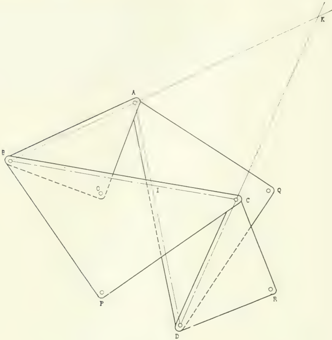
FIG. 7. QUADRUPLANE.
