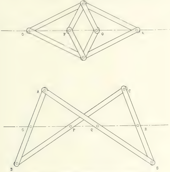
FIG. 4. HART'S CONTRA-PARALLELOGRAM.
