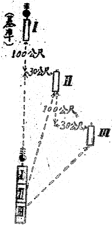
第十圖其三 梯次配置向右疏開之一例
