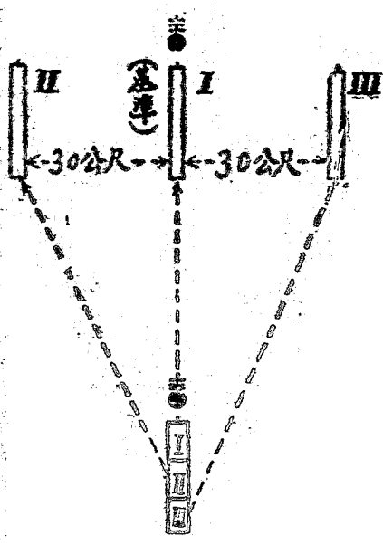
第二十圖其二 一線配置疏開之例一
