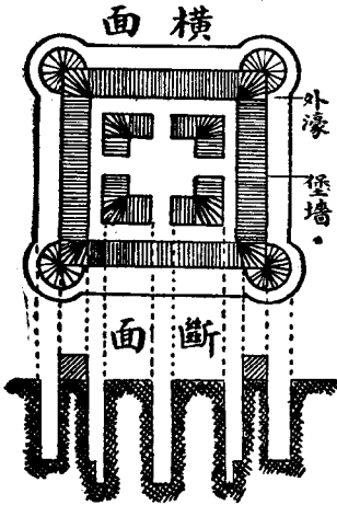
例之式圖壘碉
