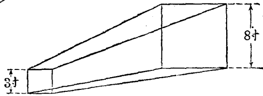
第五圖 槍眼圖
