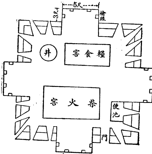
第三圖 第一層橫斷圖
