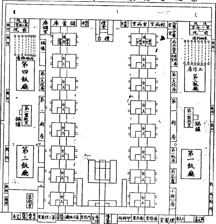
某地營房(下樓)間數全圖
