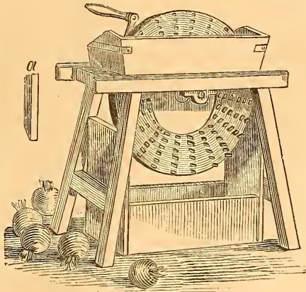
Fig. 3.—ROOT PULPER.
