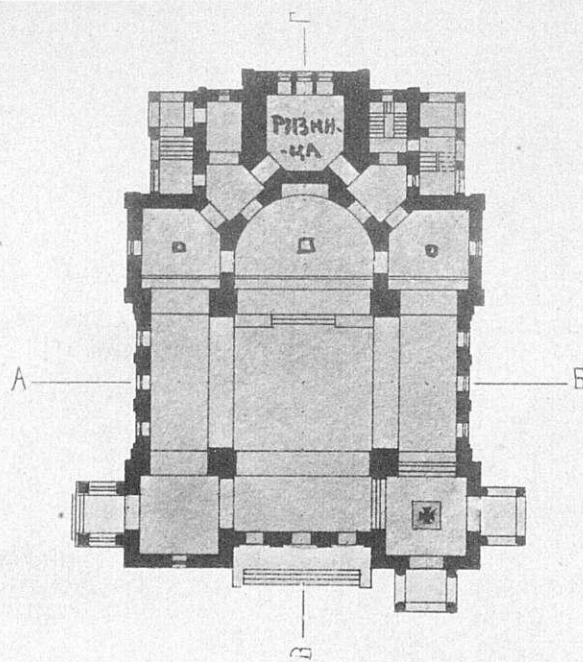
Планъ.
