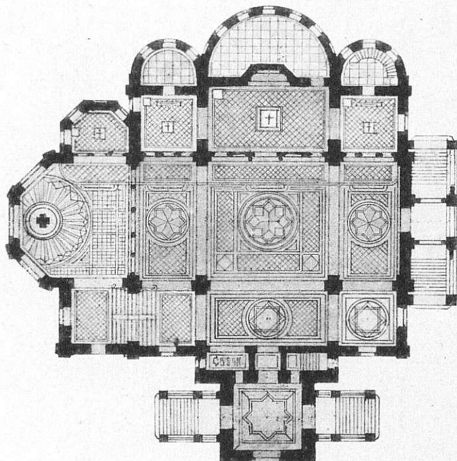
П л а н ъ.
