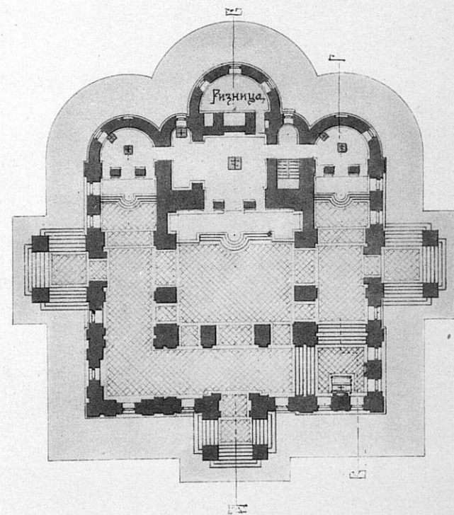
П л а н ъ.
