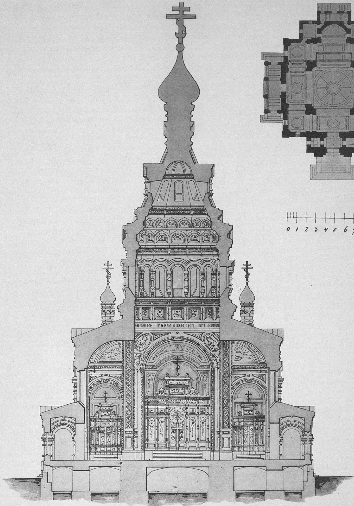
Поперечный разръзъ.
