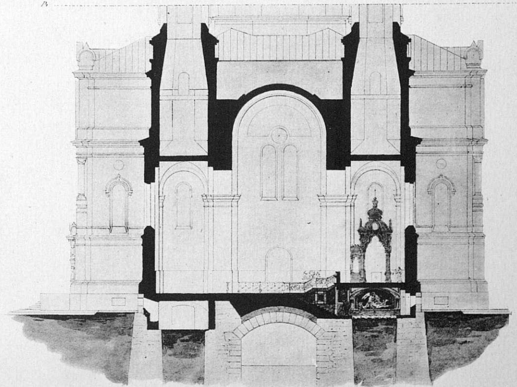
Разрѣзь по В. Г.
