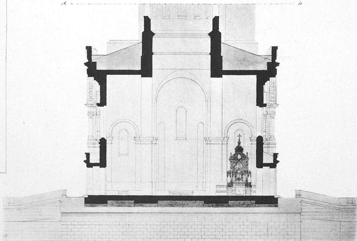
Разрѣзь по А. Б.
