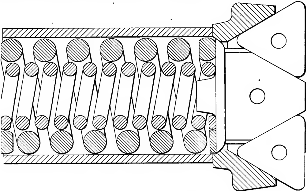
FIG. 4—SESSIONS TYPE K GEAR
