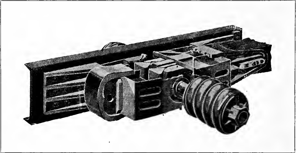
FIG. 6—CARDWELL TYPE G-25-A GEAR
