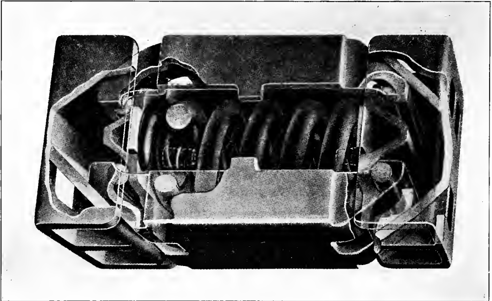
FIG. 10—MURRAY TYPE H-25 GEAR
