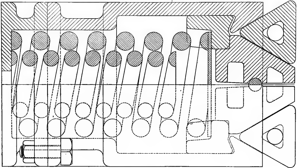
FIG. 14—CHRISTY GEAR
