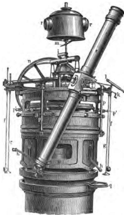
Фиг. 3. Аль азимутъ Страсбургской Обсерваторіи. Объективъ Мерца въ Мюнхенѣ, механическая часть бр. Репсольдъ въ Гамбургѣ. Діаметръ цилиндра 84 сантим., отверстіе объектива 13,3 сантим., фокусное р. расстояние 1,5 метра.
