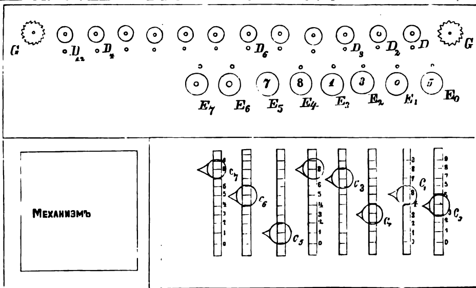
Схематическій черт. Арифмометра Томаса.
