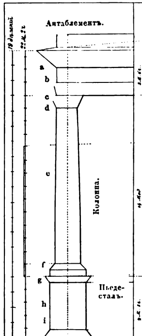
Черт. 11-й. Полный ордець.
