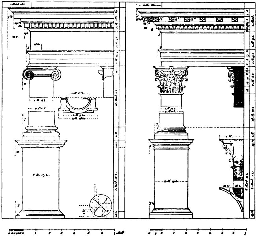
Черт. 14-й. Ионический орденъ.
