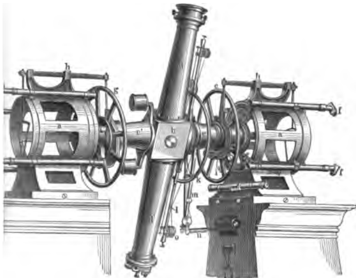
Фиг. 4. Меридіанный кругъ Страсбургской Обсерваторіи. Уровень бр. Репсольдъ въ Гамбургѣ, объективъ Мерца въ Мюнхенѣ, отверстіе объектива 16 сантим., фокусное расстояние 1,5 метровъ.
