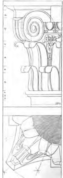
Черт. 12-й. Сложн. капит.
