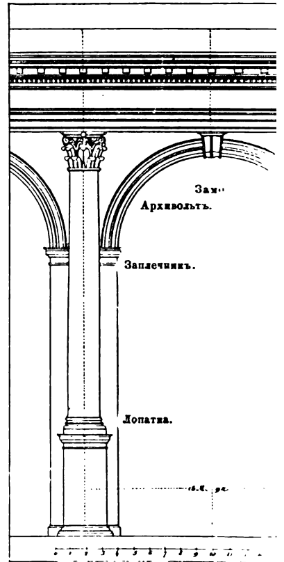
Черт. 12-й. Сложн. капит.
