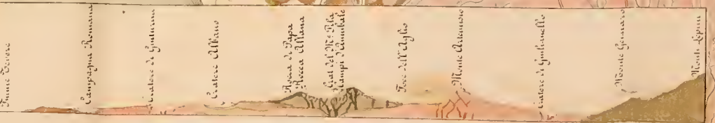
SEZIONE DEI VULCANI LAZIALI
