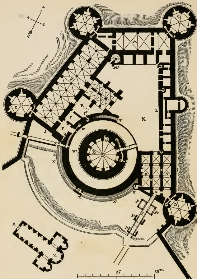
CHÂTEAU DE COUCY (Ground Plan)
