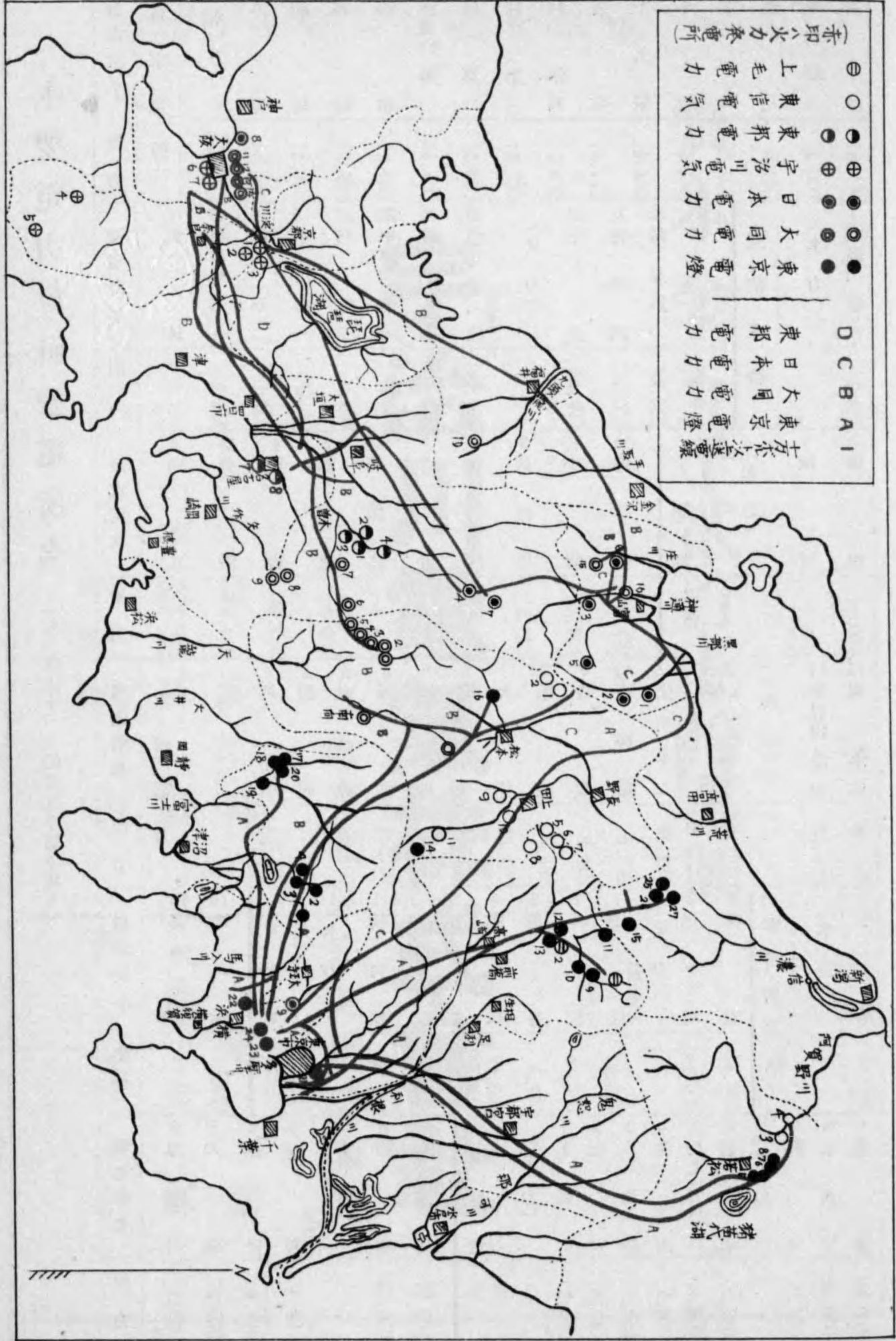
本州中北部十萬人以上送電線路圖
