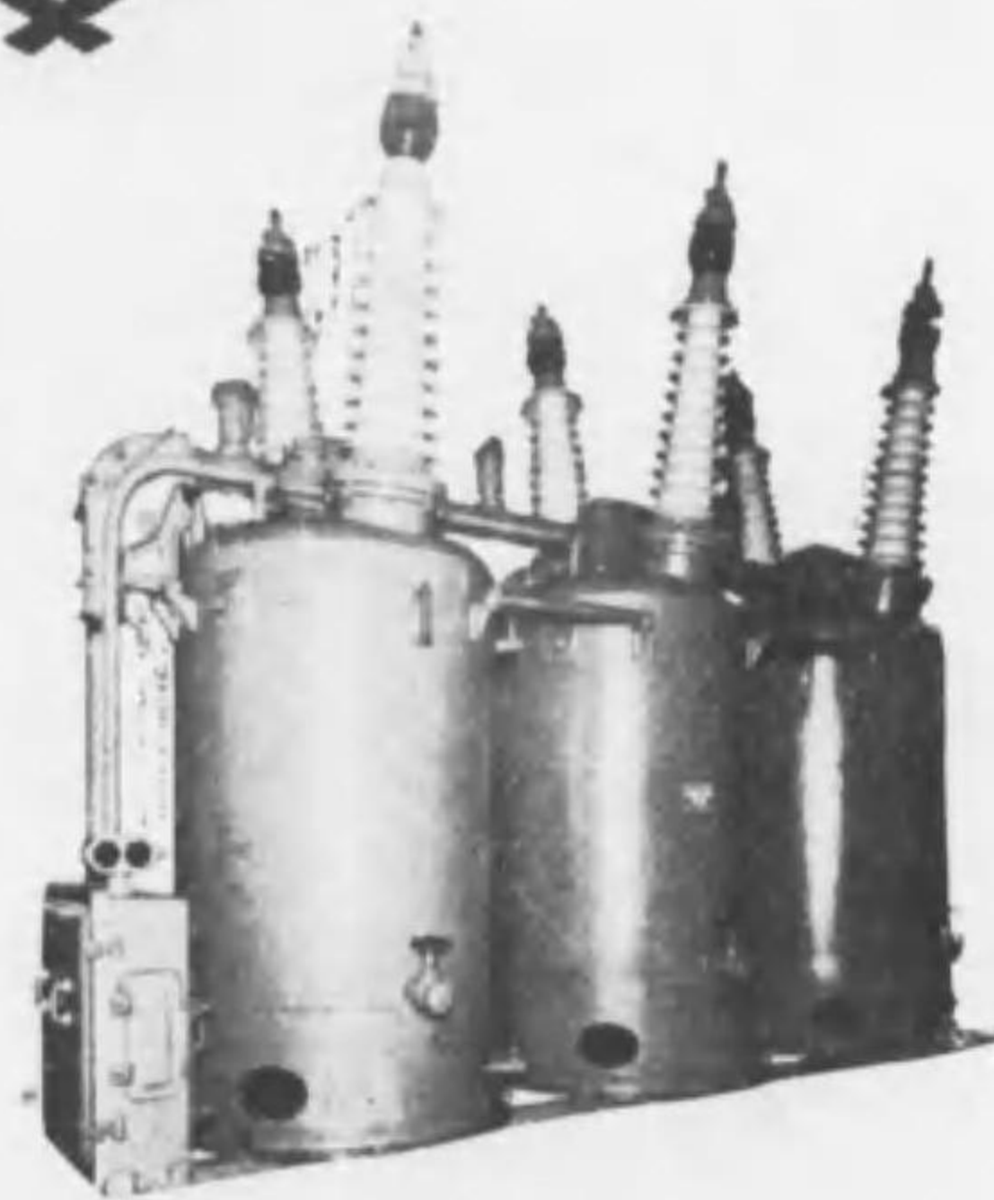
電磁操作式 屋外油入遮斷器 132KV, 600A / 100,000KVA
