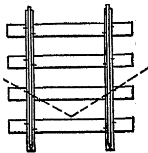
第六圖(a) 打道釘法
