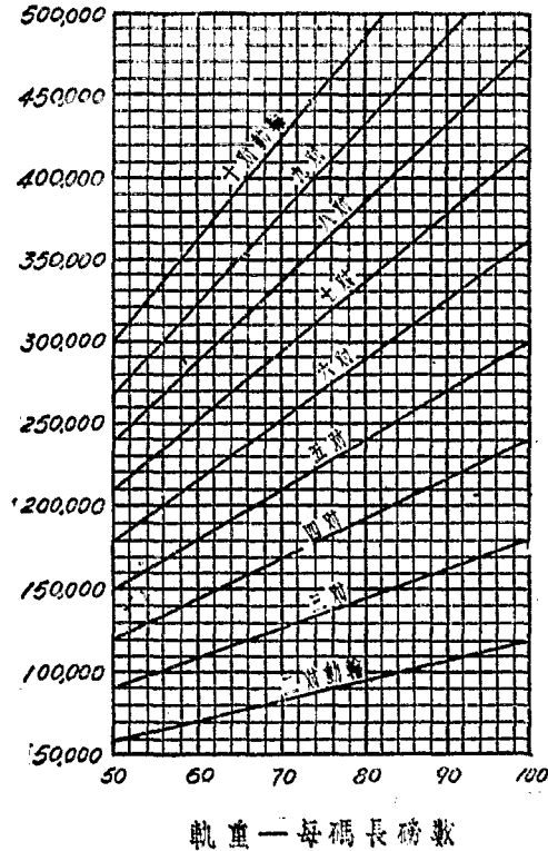
第二圖 求動輪對數曲線
