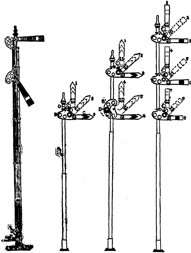
第四十六圖 二象旗號圖
