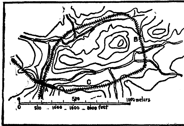
第五十三圖 橋樑繞曲環線
