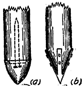
第十六圖 樁尖與樁底
