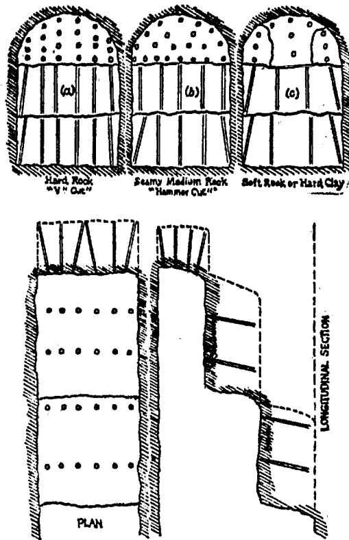
第二十七圖 鑽眼方法
