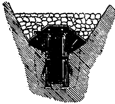
第二十九圖 洞門木架圖
