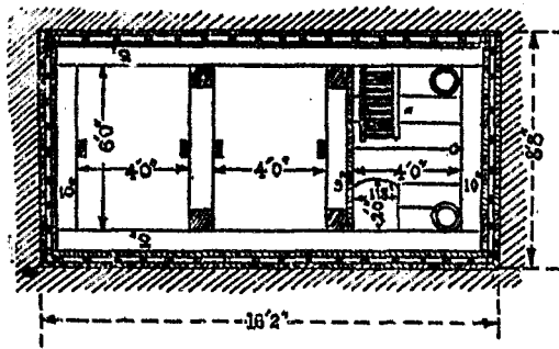
第二十三圖 直井之橫剖面圖
