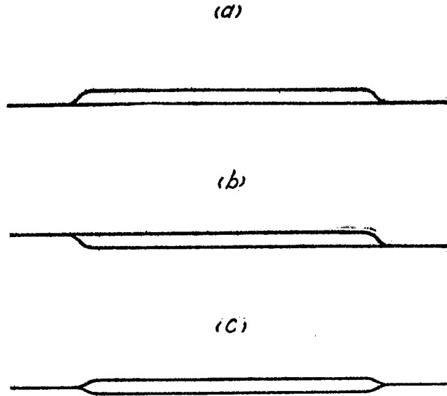
第三十六圖 避車道形式圖
