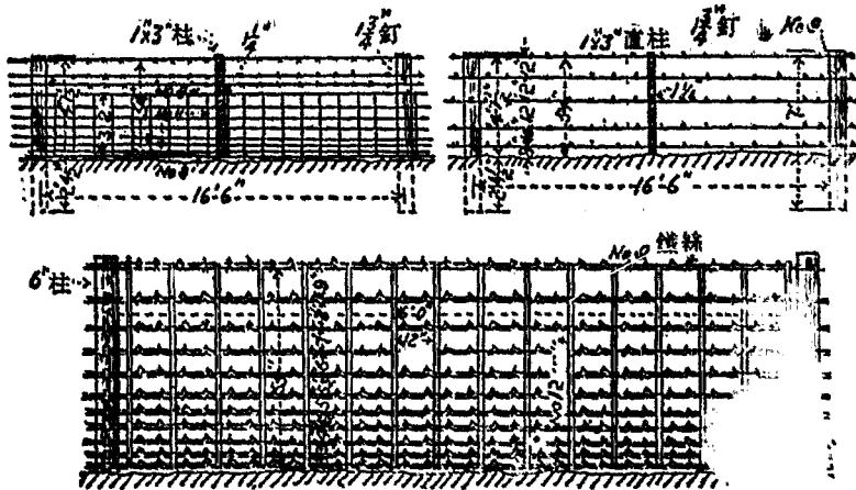
第四十二圖 路權欄
