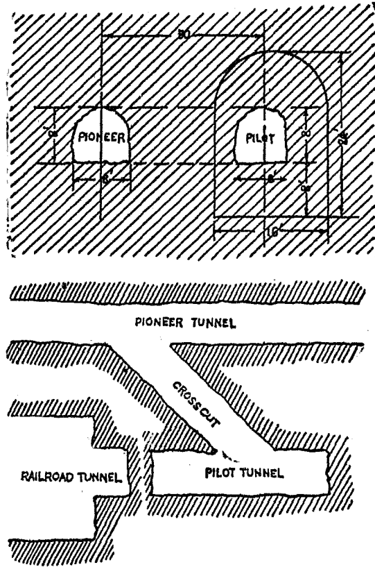
第二十八圖 先鋒及領港隧道圖
