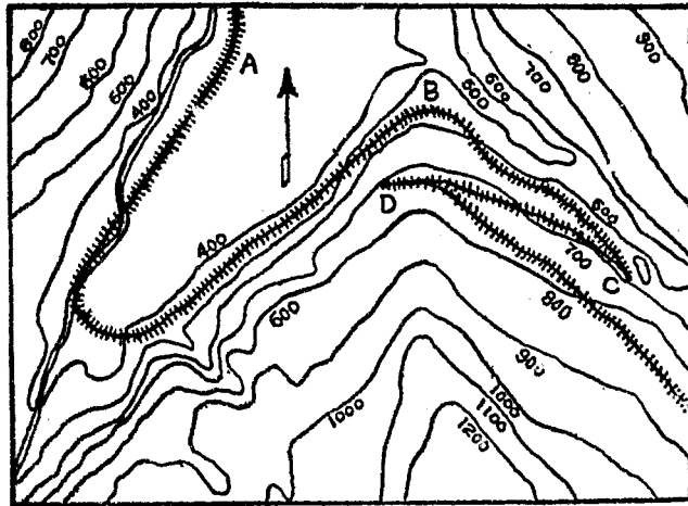
第五十二圖 迂迴線
