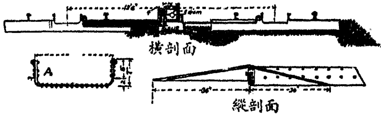
第三十九圖 軌池
