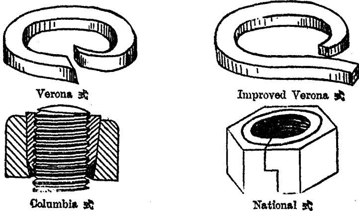
第五圖 螺釘帽鎖式樣
