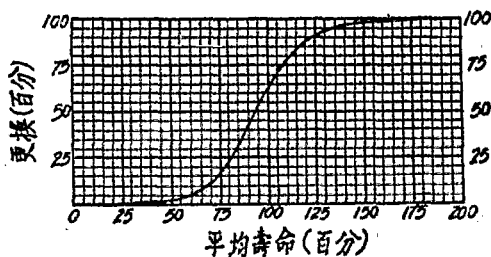
第八圖 枕木之相關真壽命
