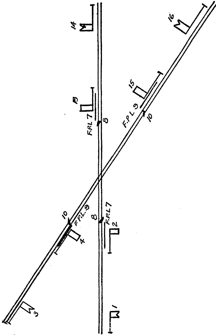
第五十圖 平交連鎖圖
