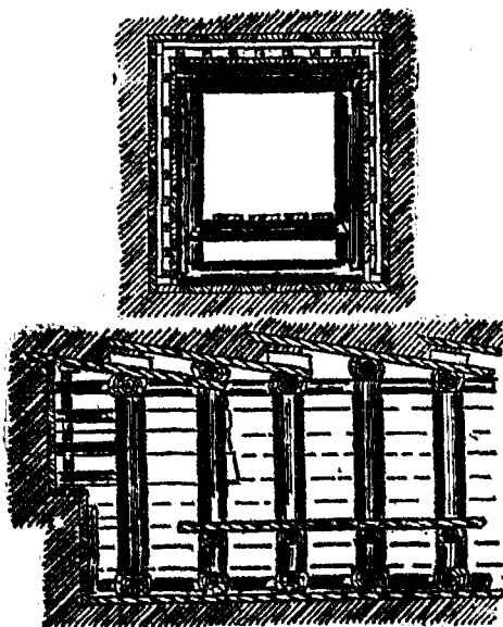
第二十五圖 導坑木架圖
