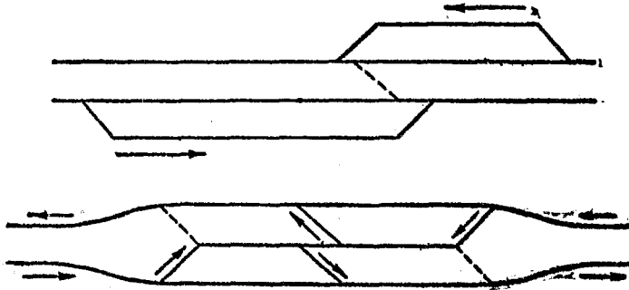
第三十二圖 副路佈置圖
