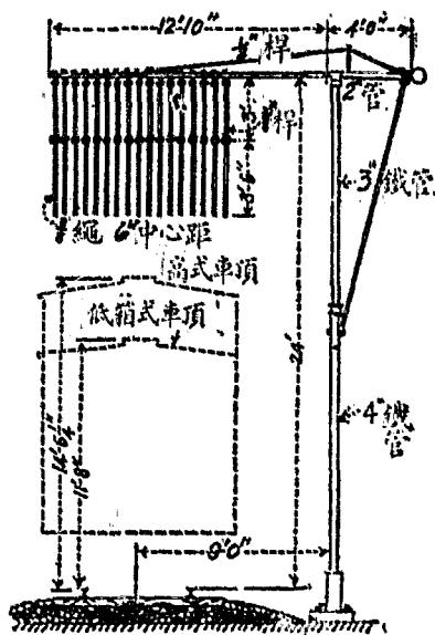
第四十三圖 橋樑警告標
