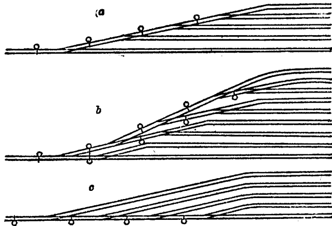
第三十三圖 梯軌式樣圖
