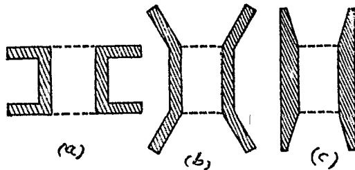
涵洞之樣式
