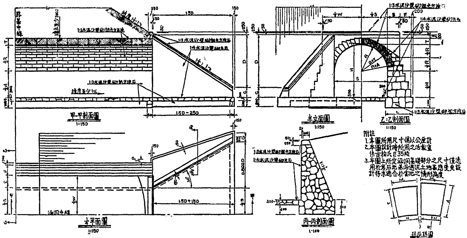
第十三圖 (d) 演繹路石砌拱形涵洞標準圖
