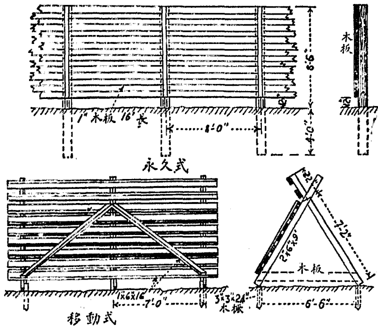
第四十圖 雪棚
