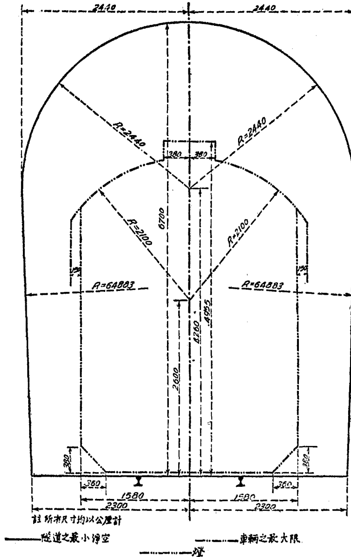
第二十圖(a) 單線隧道之最小淨空
