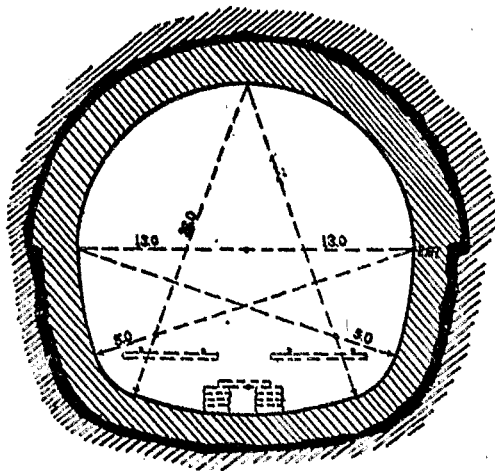
第二十二圖 隧道橫剖面圖
