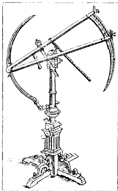
第十三圖 第谷天文六分儀 (鋼製，臂 AB 及 AC 長凡四英尺)
