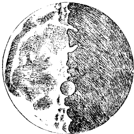
第二十五圖 加里尼 所給月面影像草圖
