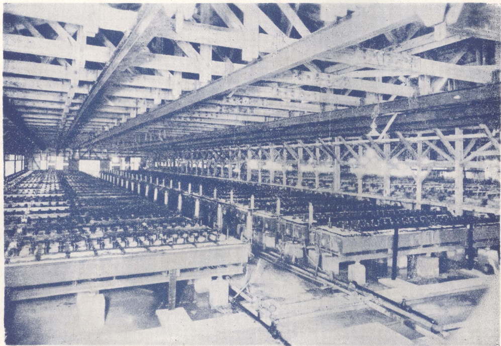
(6) 隔膜式電解槽
