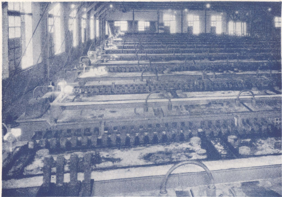
(7) 水銀電解槽
