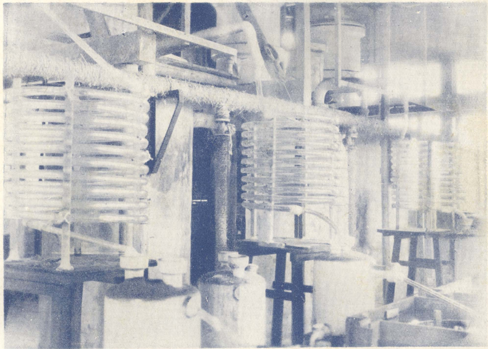
(14) 溴素蒸溜工場
