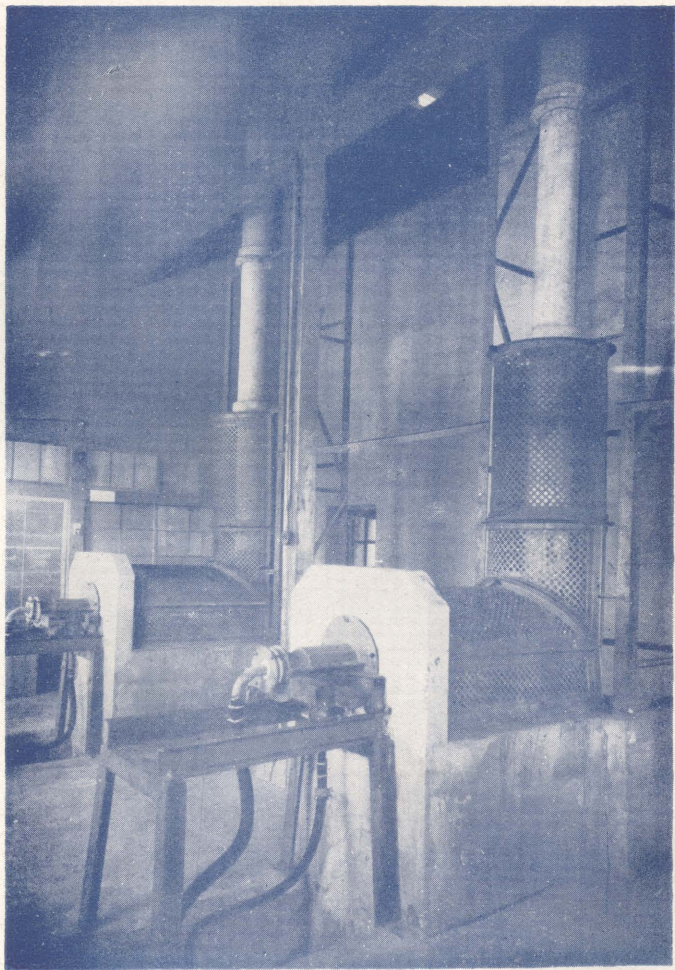
(11) 鹽酸合成塔
