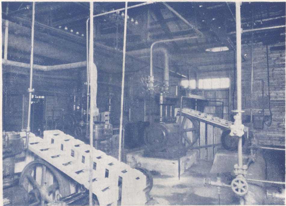
(10) 液 氣 工 場
