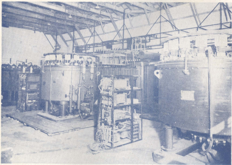
(5) 水銀整流器
