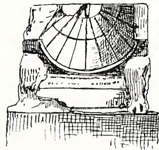
Cadran solaire des thermes de Stabies.
