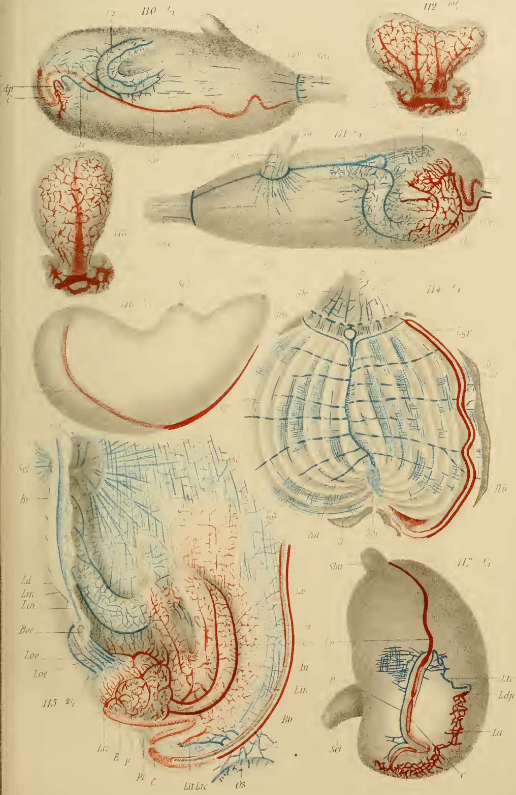
Circulation des Cynthadées.
