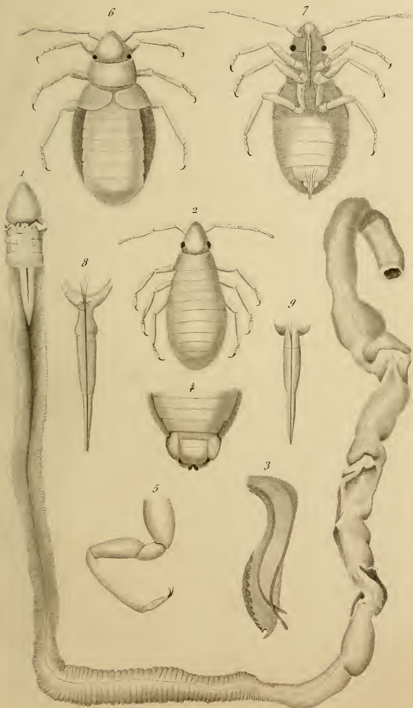
1. Balanoglossus sarniensis . — 2 à 9 Epophilus Bonnairei .
