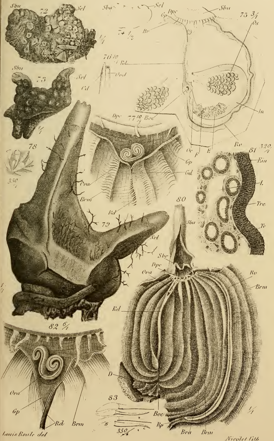
Cynthia panter , Microcosmus vulgaris .
