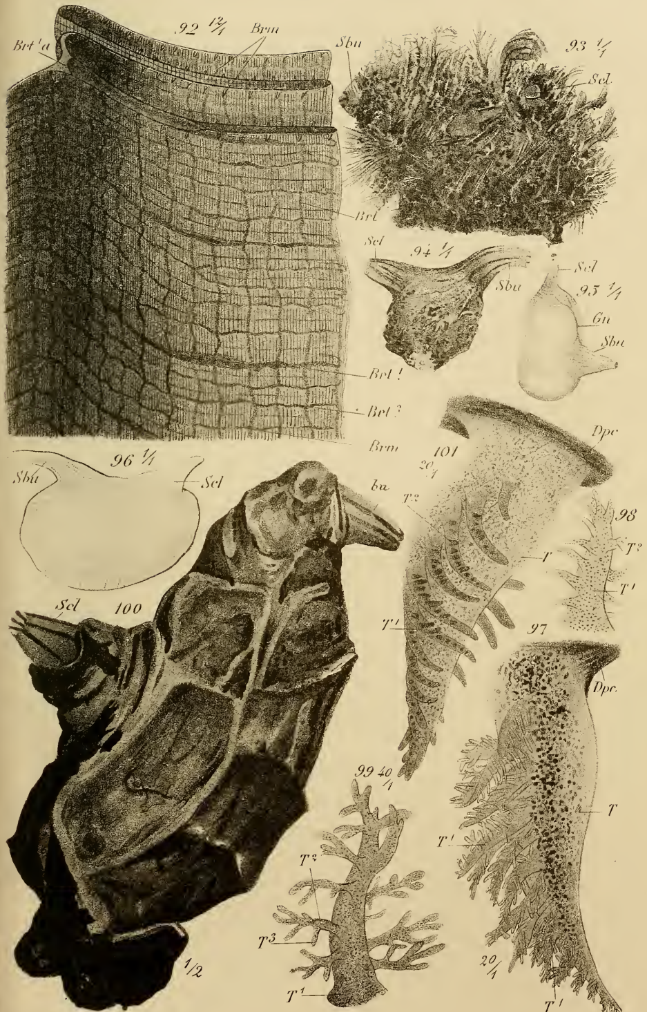
Microcosmus Vulgaris, M. Sabatieri, M. Polymorphus.
