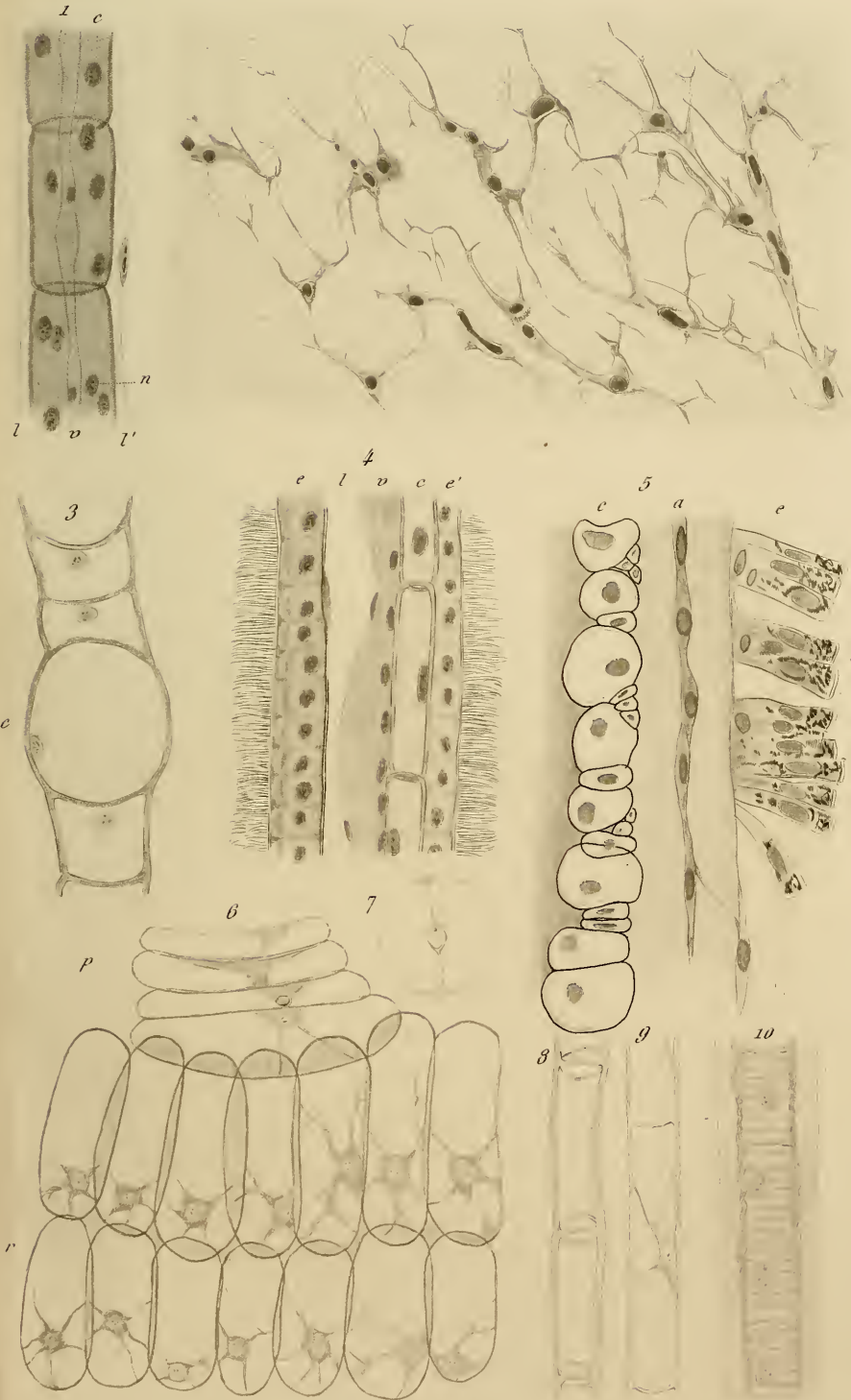
Squelette branchial de la Sabelle.
