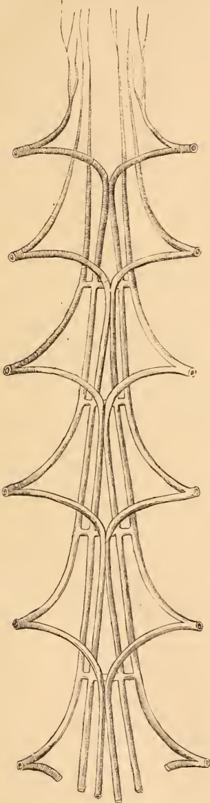
Fig. 41. Tracheæ of Geophilus subterraneus , \times 140 .
