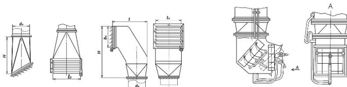
Тип УДВ - с увлажнением воздуха (для адиабатического охлаждения)
