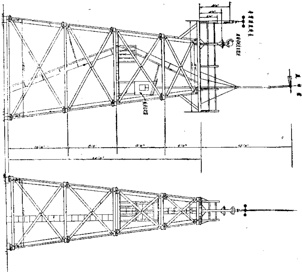
塔身正面圖
