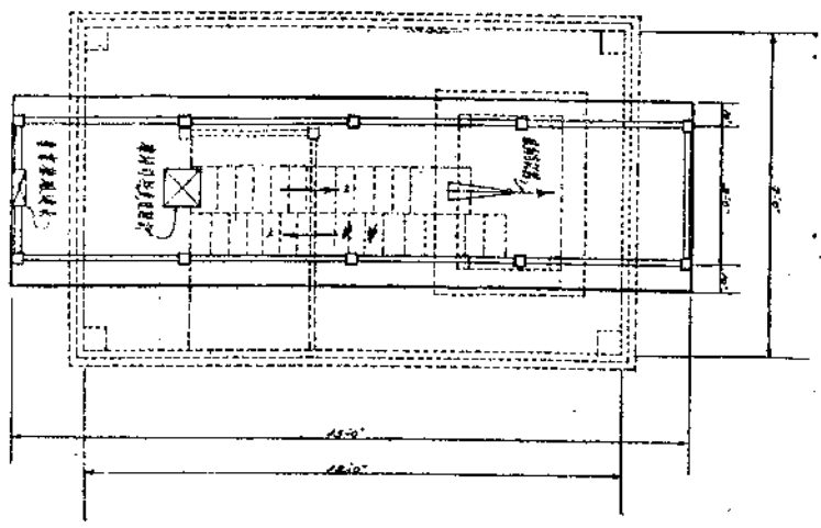
塔身第二層平面圖
