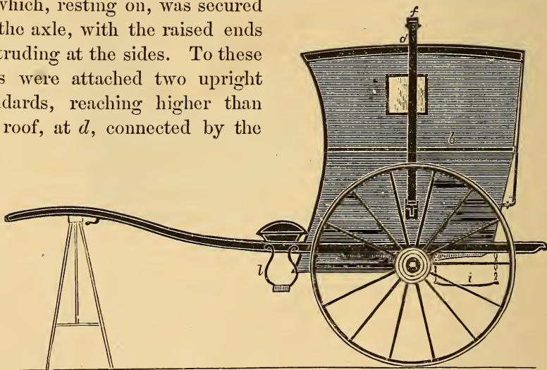
AVRIL'S TRIOLET.
