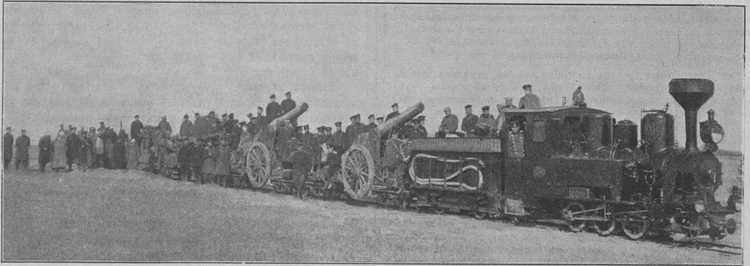
Двѣ 6-ти-дюймовыя пушки, привезенныя на вагонеткахъ по военно-полевой желѣзной дорогѣ на конечный пунктъ — 27-я верста отъ Люблина, на станцію Косержевъ, для установки ихъ на временно построенную осадную батарею.
