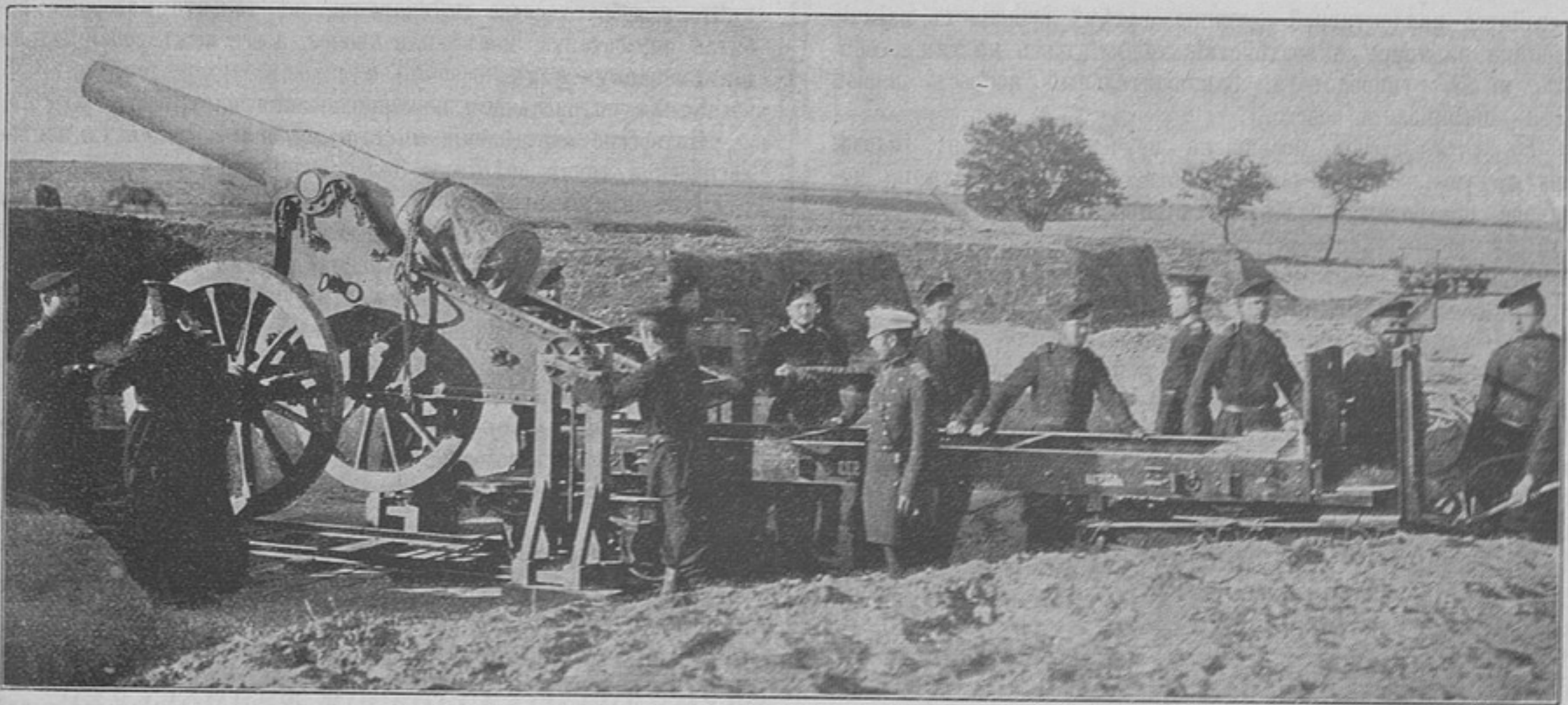
Вытягиваніе тѣлѣжки изъ-подъ 6-ти-дюймовой второй пушки.
