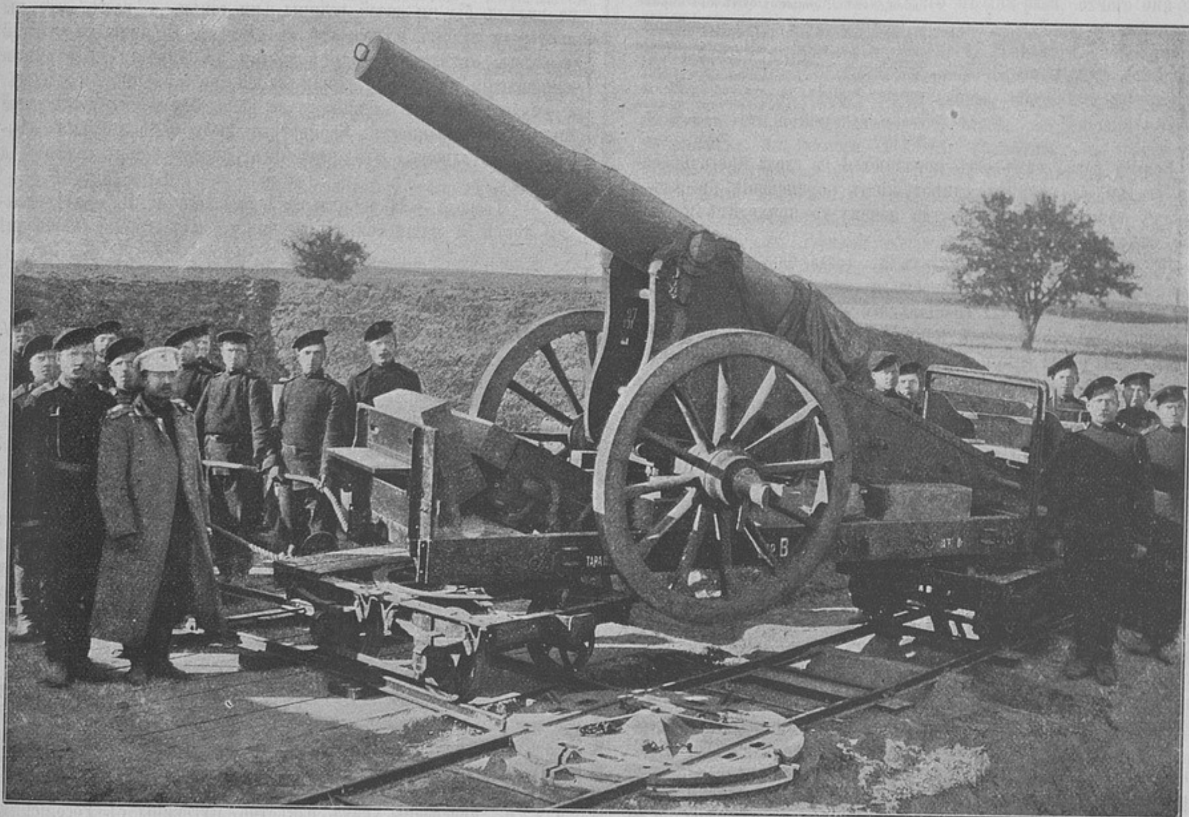
Постановка на платформу осаднаго укрѣпленія первой 6-ти-дюймовой пушки, при поворотѣ на пути 90°.
