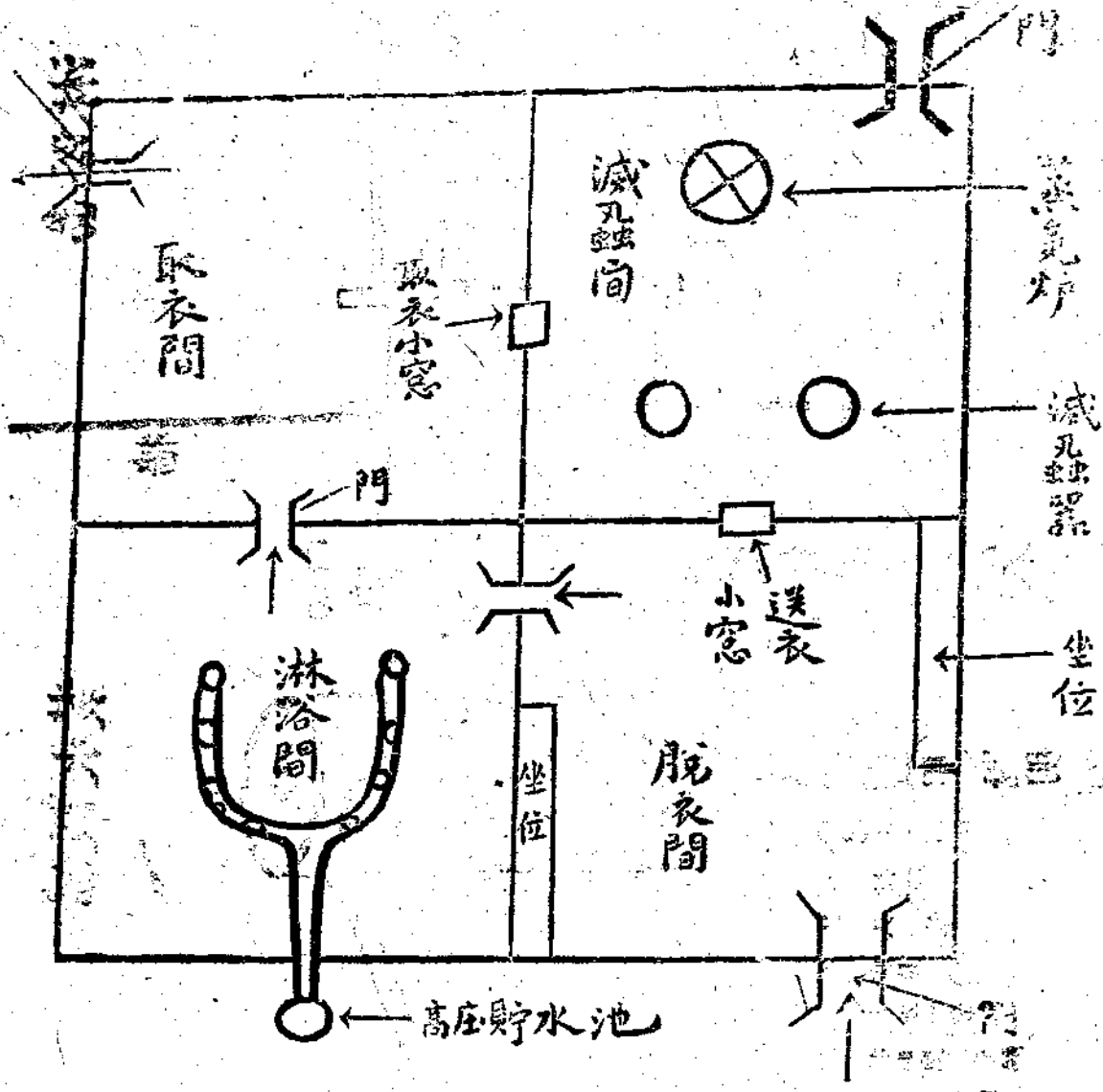
淋浴及滅虱間圖(乙)
