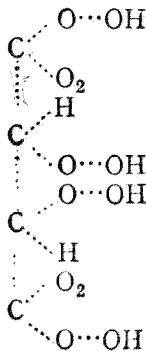
酒石酸
