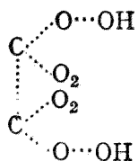
草酸
