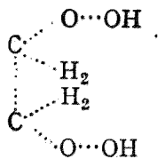
乙二醇 (glycol)
