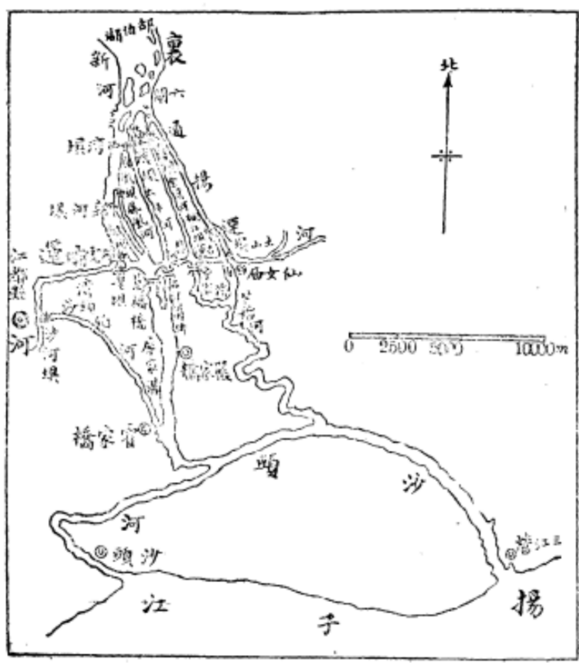
圖三 揚子江歸河運渠各壩總圖
