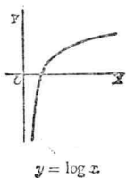
對數曲線 LOGARITHMIC CURVE
