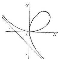
笛卡兒之蚌線 FOLIUM OF DESCARTES
