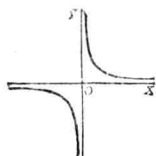
等邊雙曲線 EQUILATERAL HYPERBOLA
