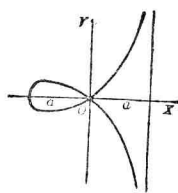
環索線 STROPHOID
