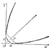
拋物線 PARABOLA
