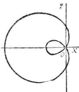
蠟線 LIMACON
