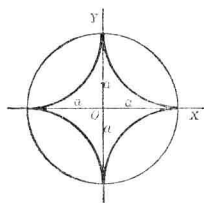
四歧点之內旋輪線 HYPOCYCLOID OF FOUR CURVES
