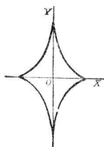
橢圓之縮閉線 EVOLUTE OF ELLIPSE
