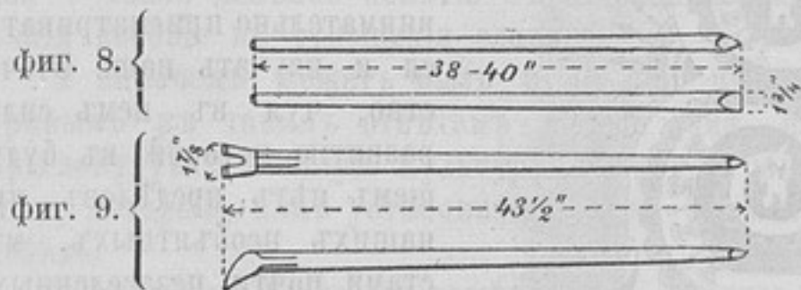
Главные нормальные размѣры ломовъ:
