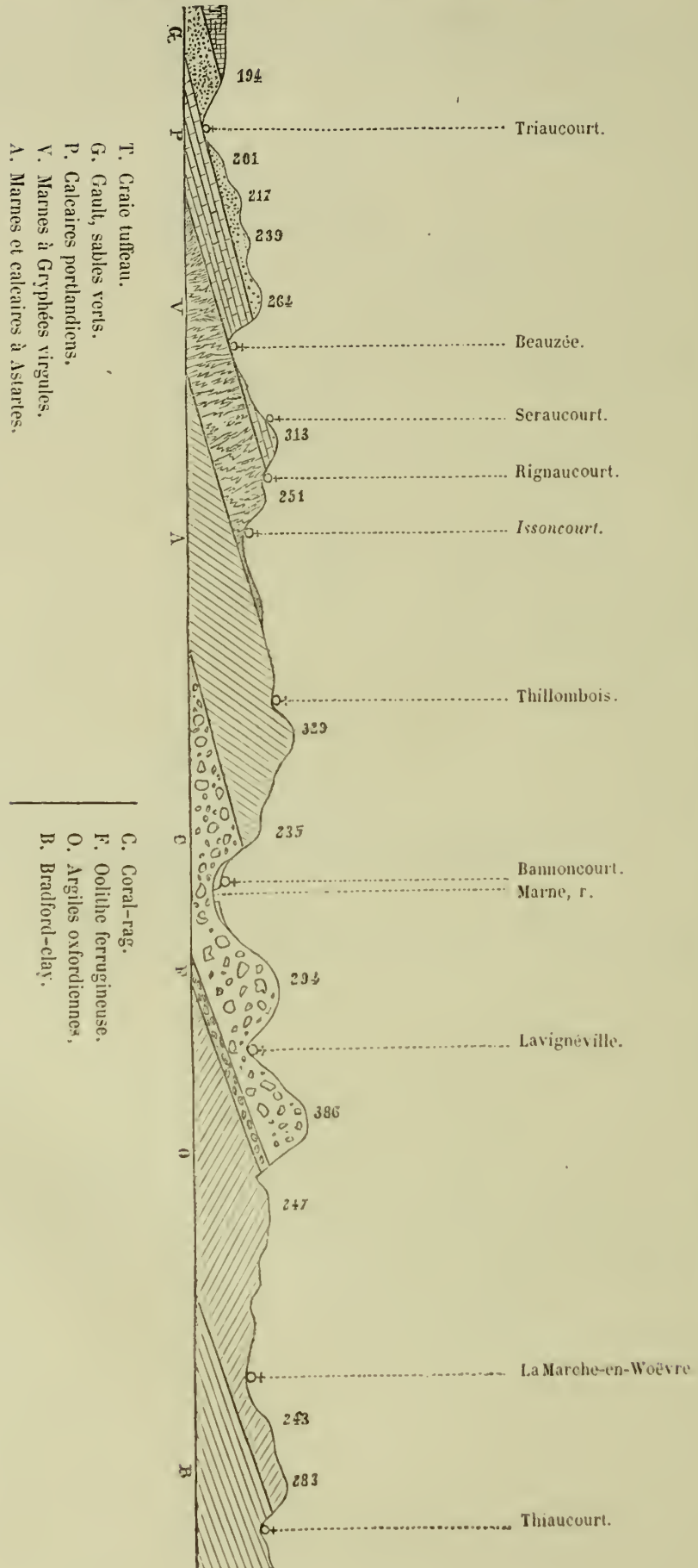
Coupe géologique traversant le département de la Meuse, de Triaucourt à Thiaucourt, par Issoncourt.
